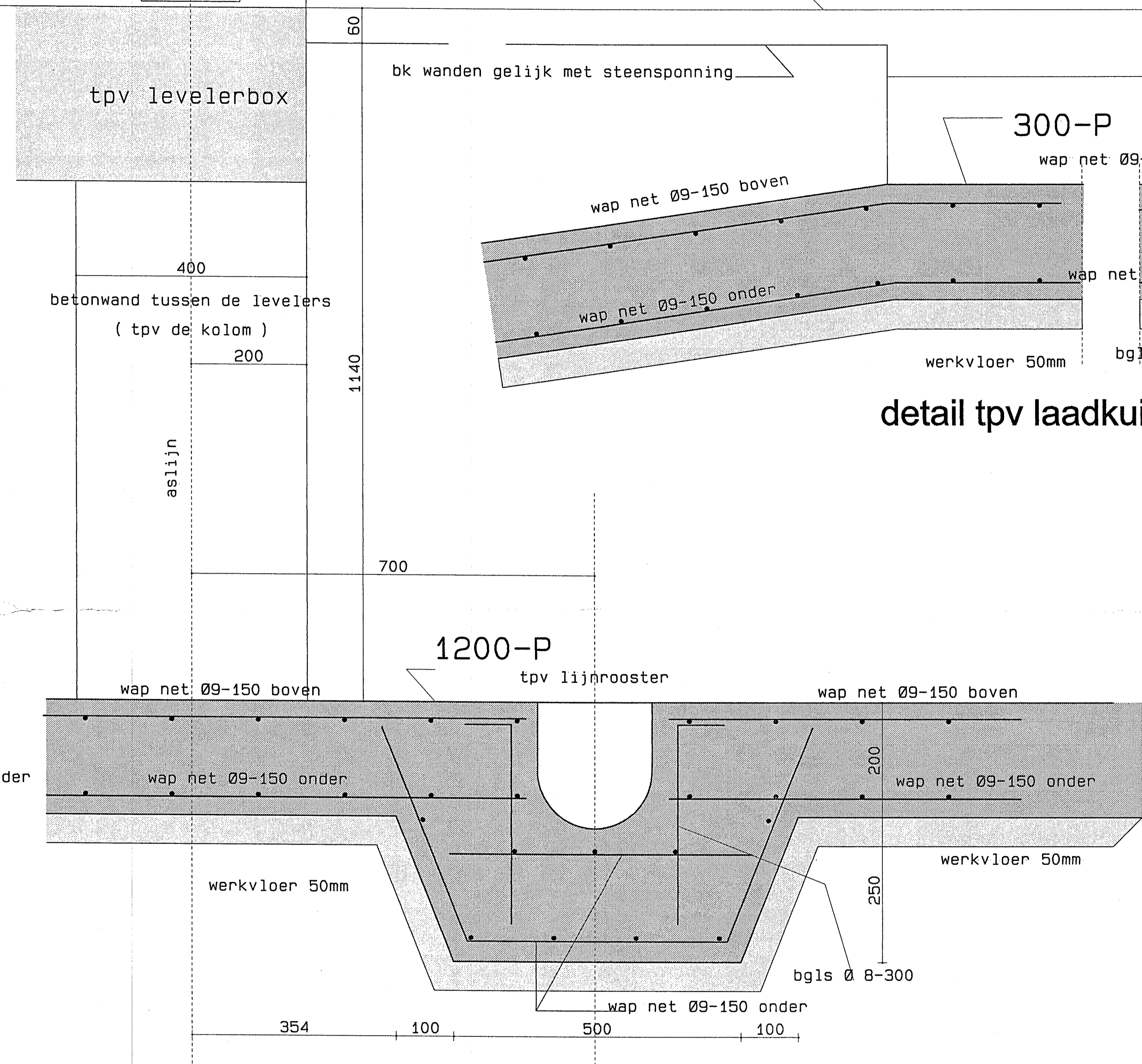
detail tpv laadkuil/lijnrooster
