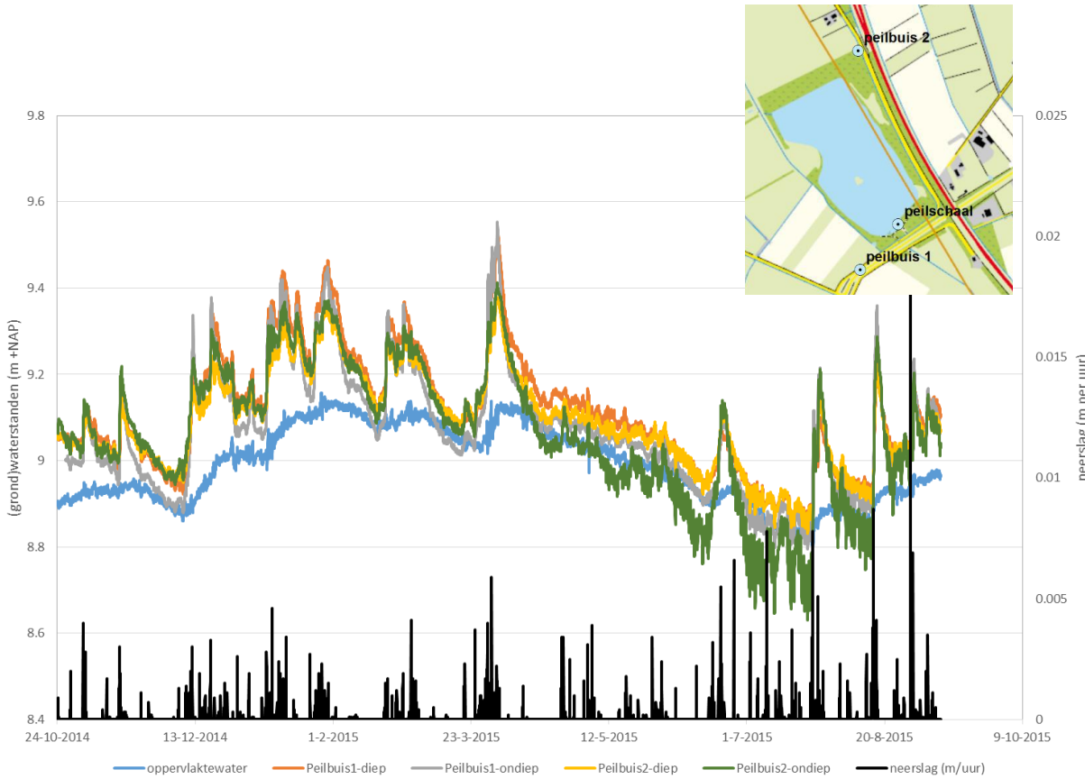
Figuur 2.3: Gemeten stijghoogten, oppervlaktewaterpeil en neerslag [Grontmij, 2015]
