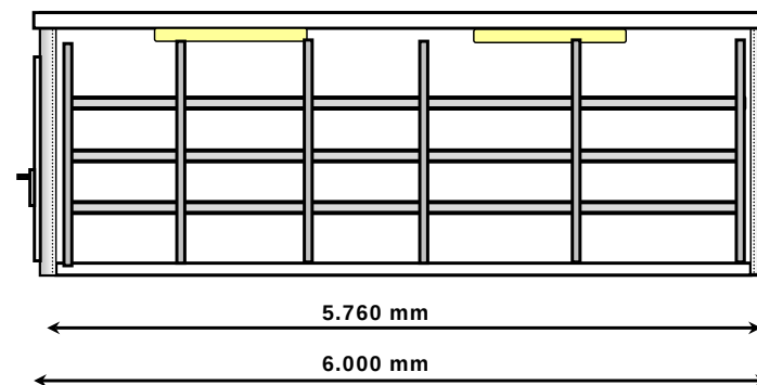
Doorsnede zij-aanzicht
