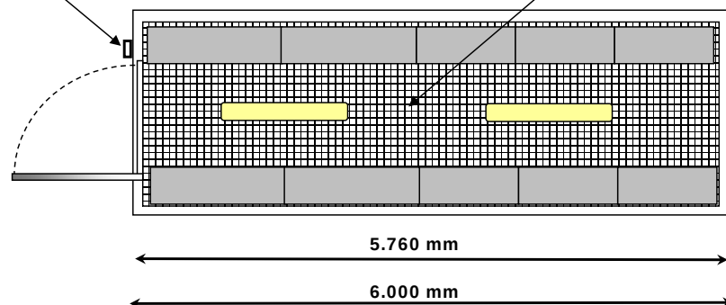
Doorsnede bovenaanzicht
