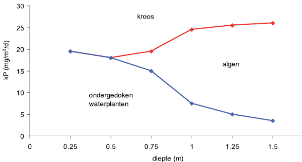
Afbeelding 3. Kritische fosfaatbelasting in sloten in relatie tot de waterdiepte bij een stroming van 50mm/d (maat voor de verblijftijd, hoe hoger de hydraulische belasting hoe korter de verblijftijd) (W+B, 2009)
