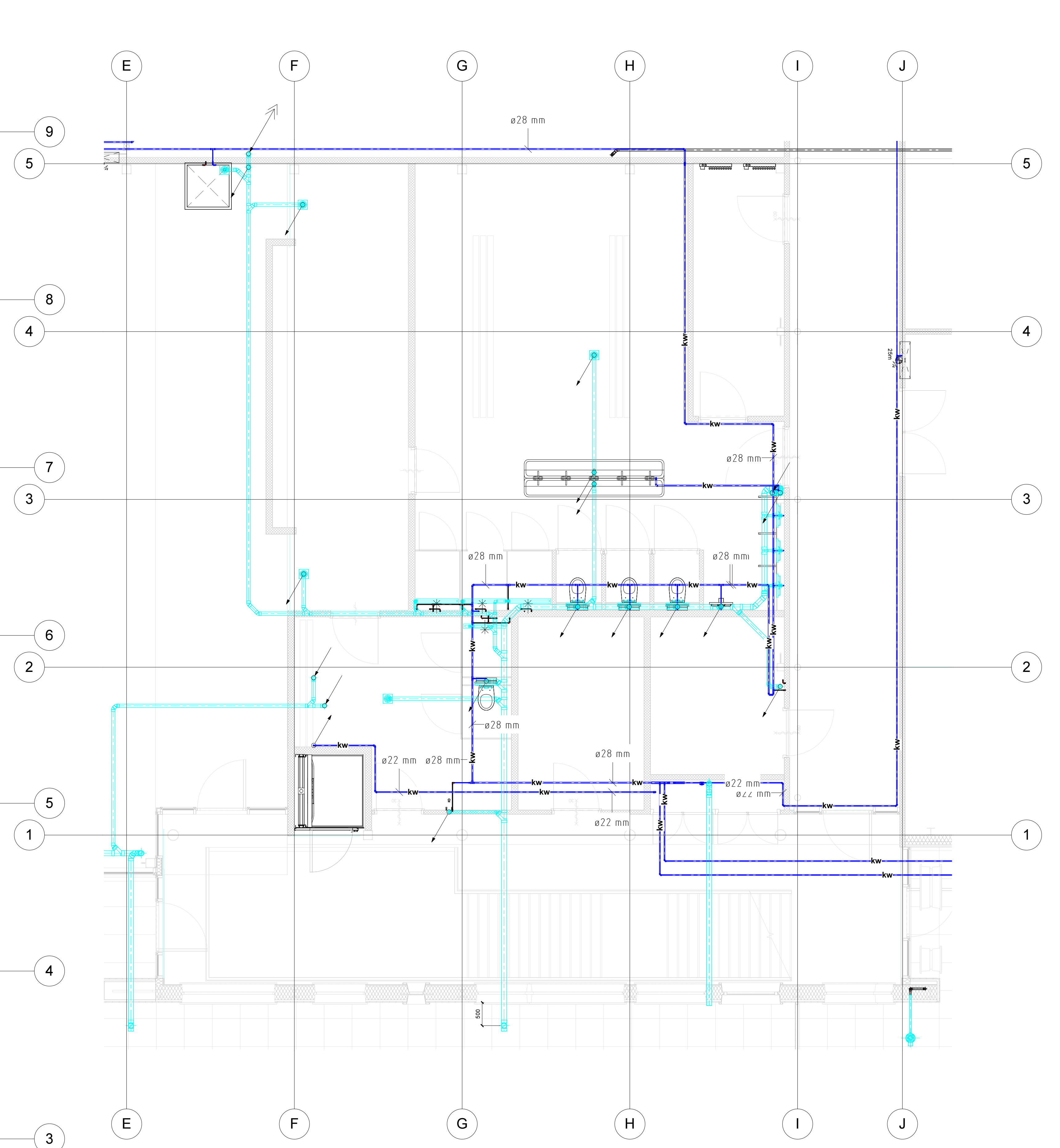
Nattegroepen begane grond 1 : 50
