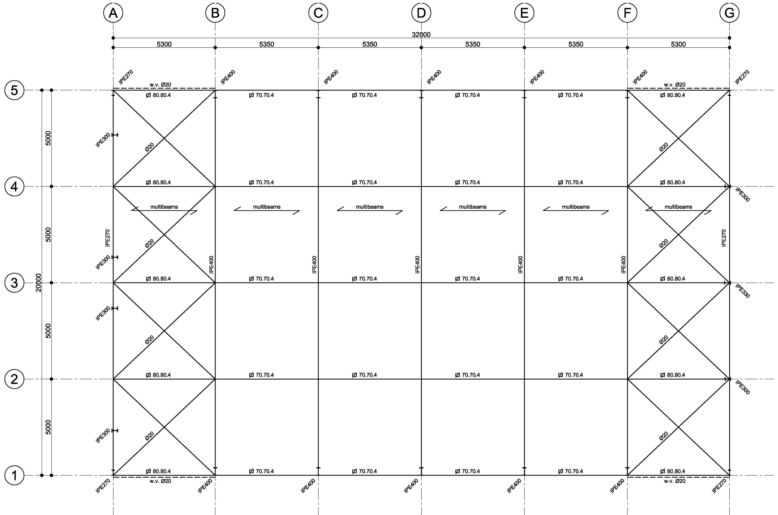
BOVENAANZICHT STAAL
