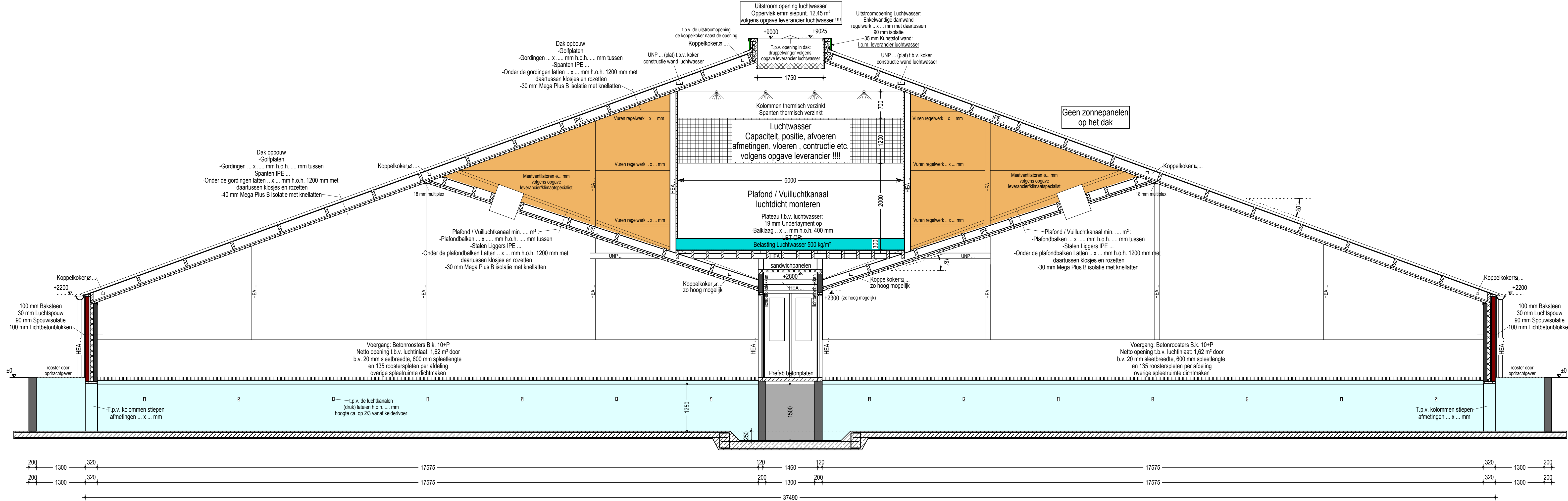
Doorsnede A-A
