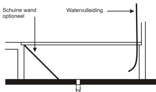
Doorsnede A-A
