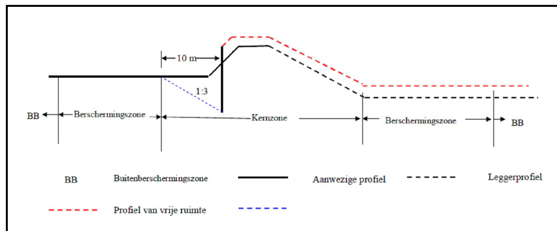
Figuur 6. Leggerprofiel en profiel van vrije ruimte van een damwand constructie
