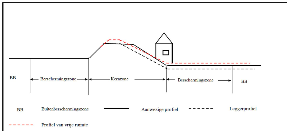
Figuur c: Leggerprofiel en het profiel van vrije ruimte van keringen met binnendijkse bebouwing
