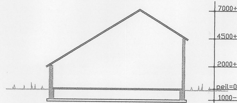
doorsnede stal 2
