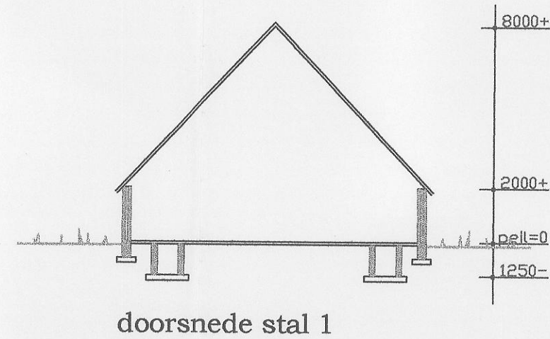
doorsnede stal 1
