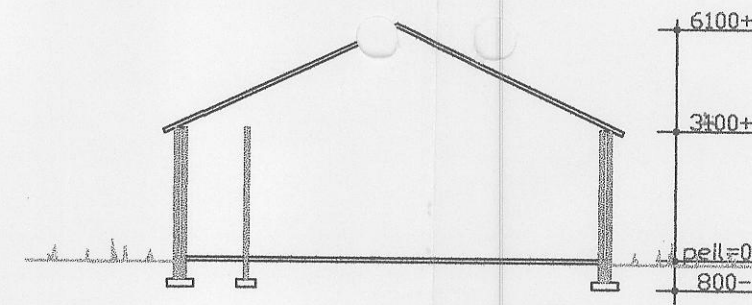
doorsnede stal 5
