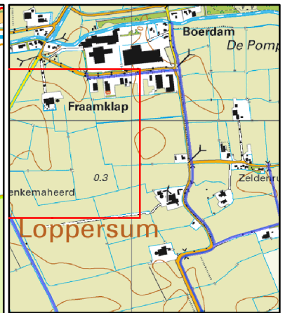
Overzicht schaal 1:25.000
