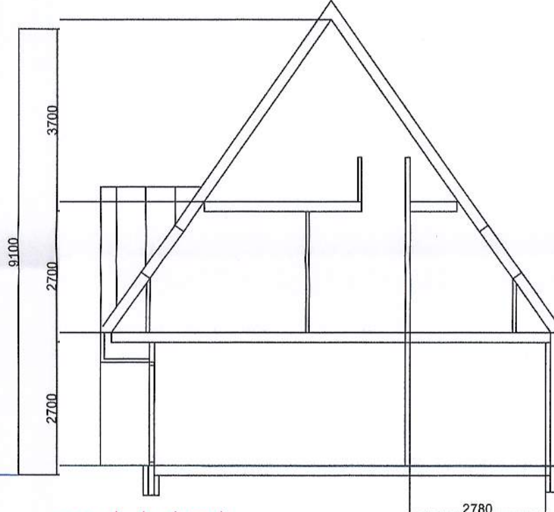
doorsnede bestaand
