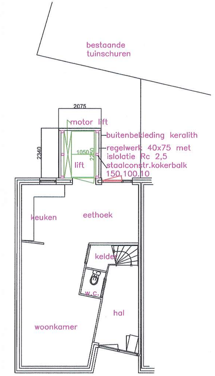
plattegrond, nieuwe toestand
