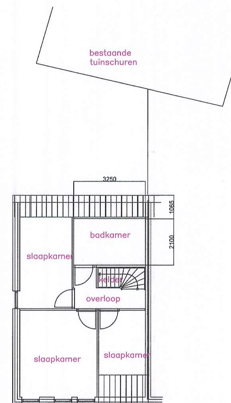
verdieping, bestaande toestand
