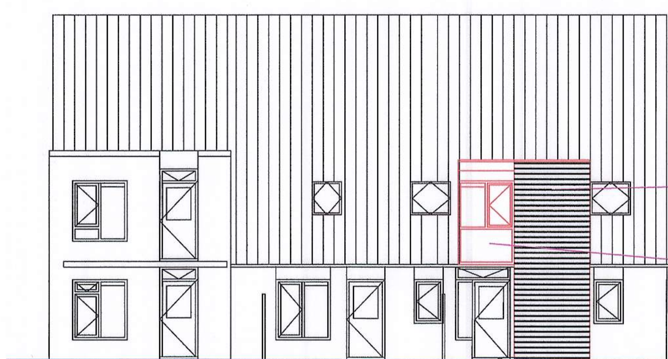
Achtergevel, nieuw
