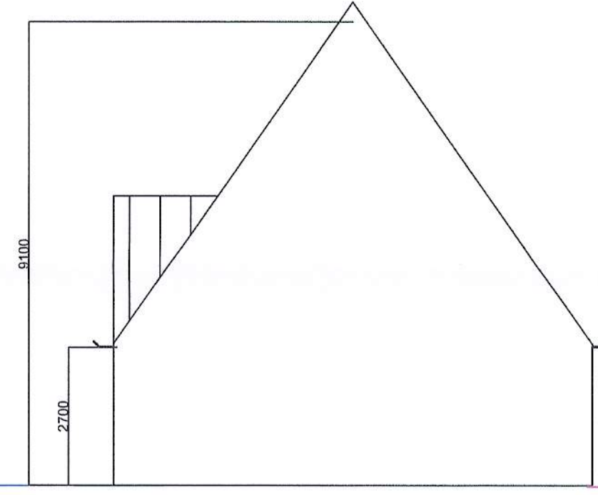
zijgevel bestaand
