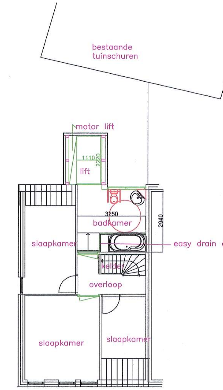
verdieping, nieuwe toestand
