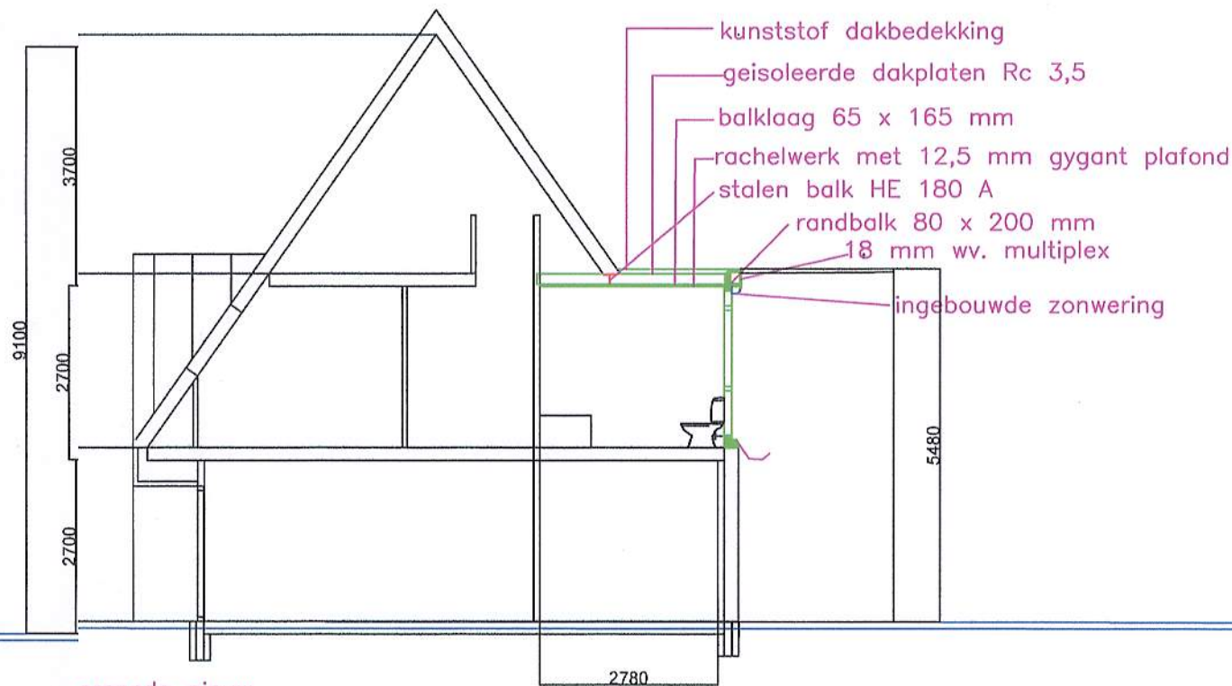
doorsnede nieuw
