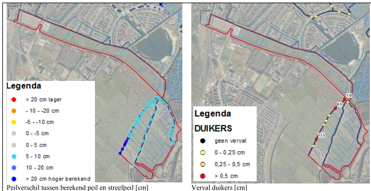
Figuur 5.26: resultaten hydraulische toetsing Oude Spaarndammerpolder
