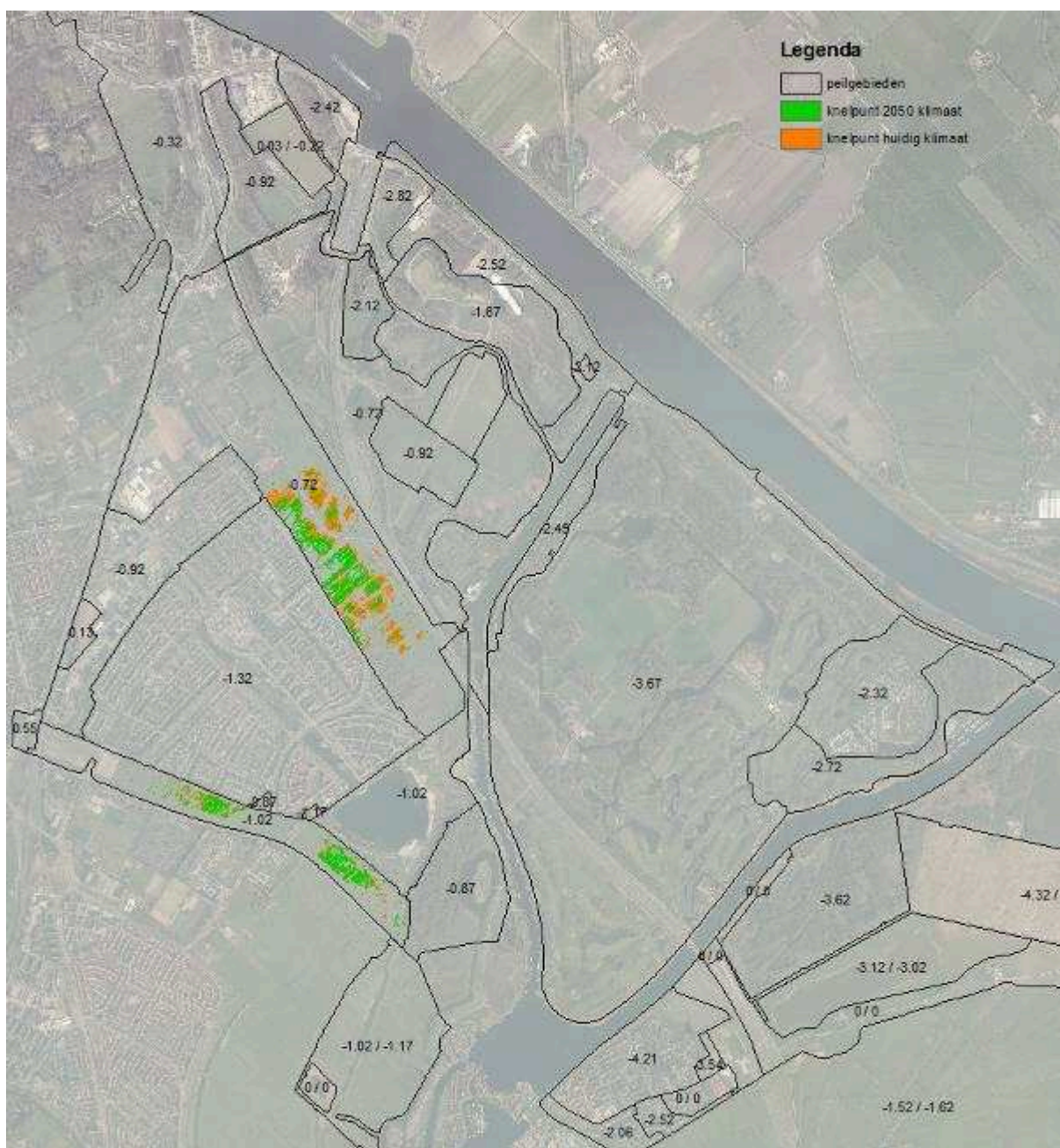
Figuur 5.31: wateroverlast huidig (oranje) en toekomstig klimaat (groen) cluster 2
