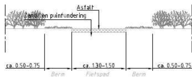
Profiel 03
