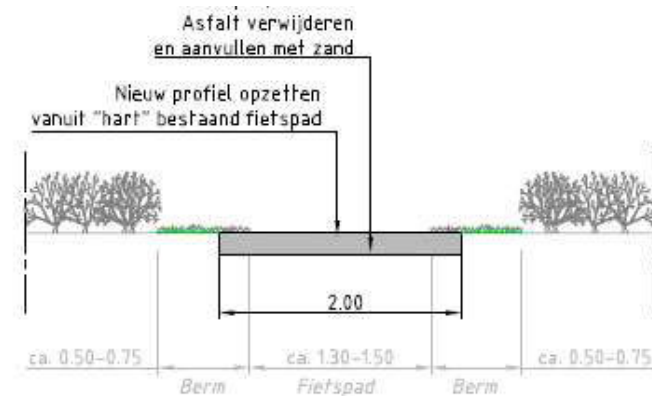
Profiel 03
