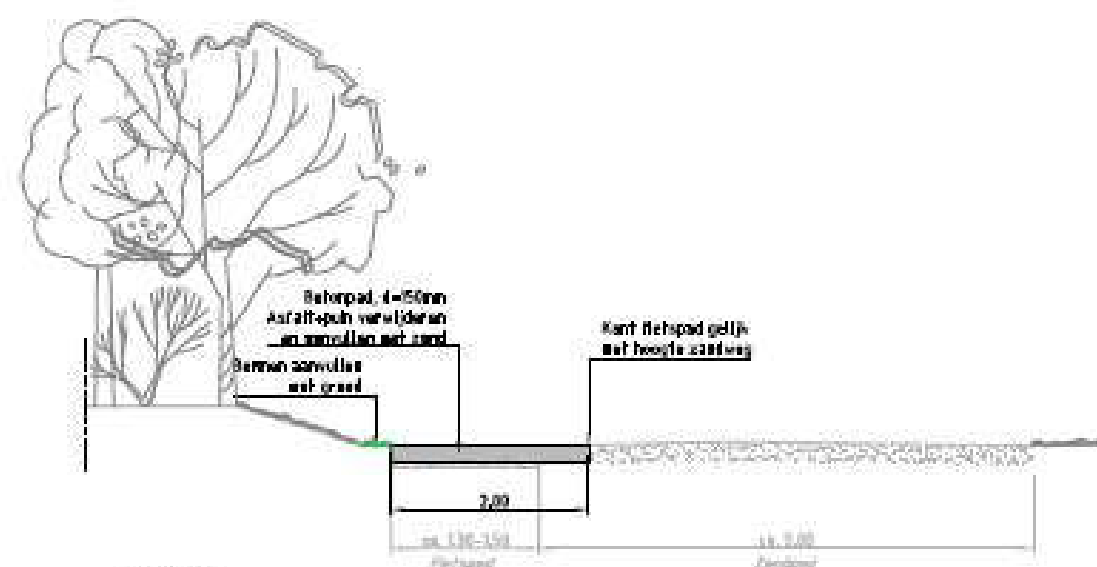
Profiel 01
