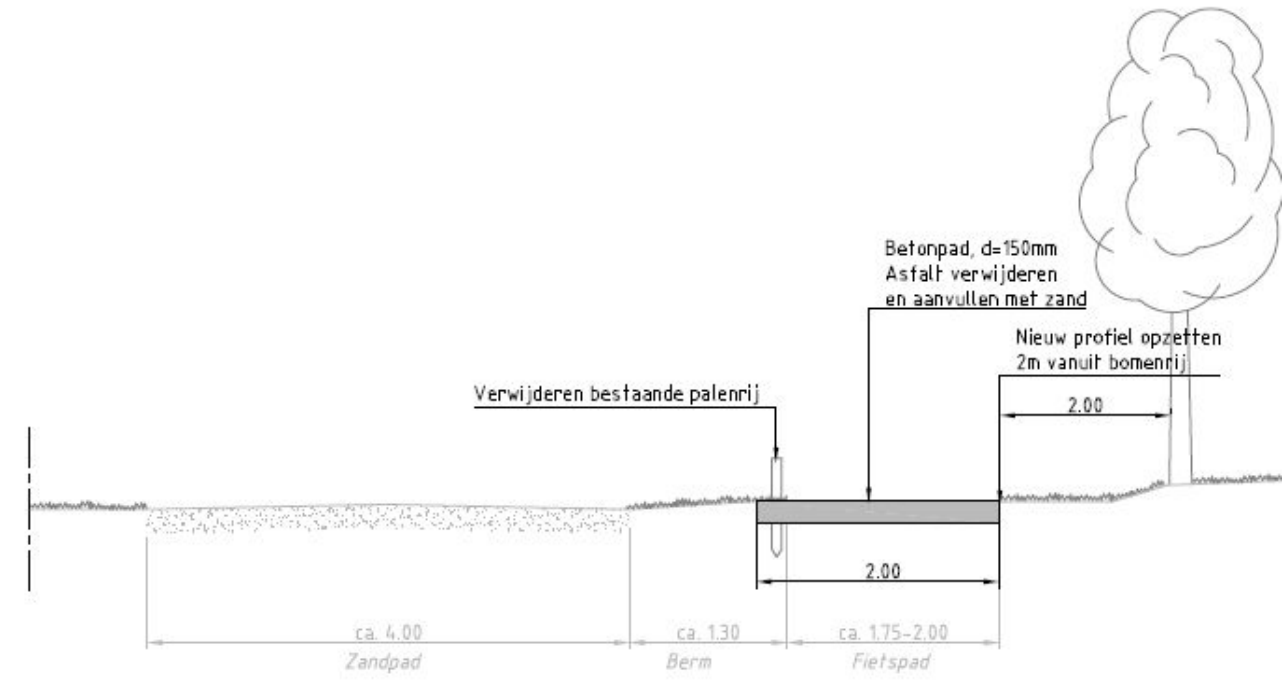
Profiel 06
