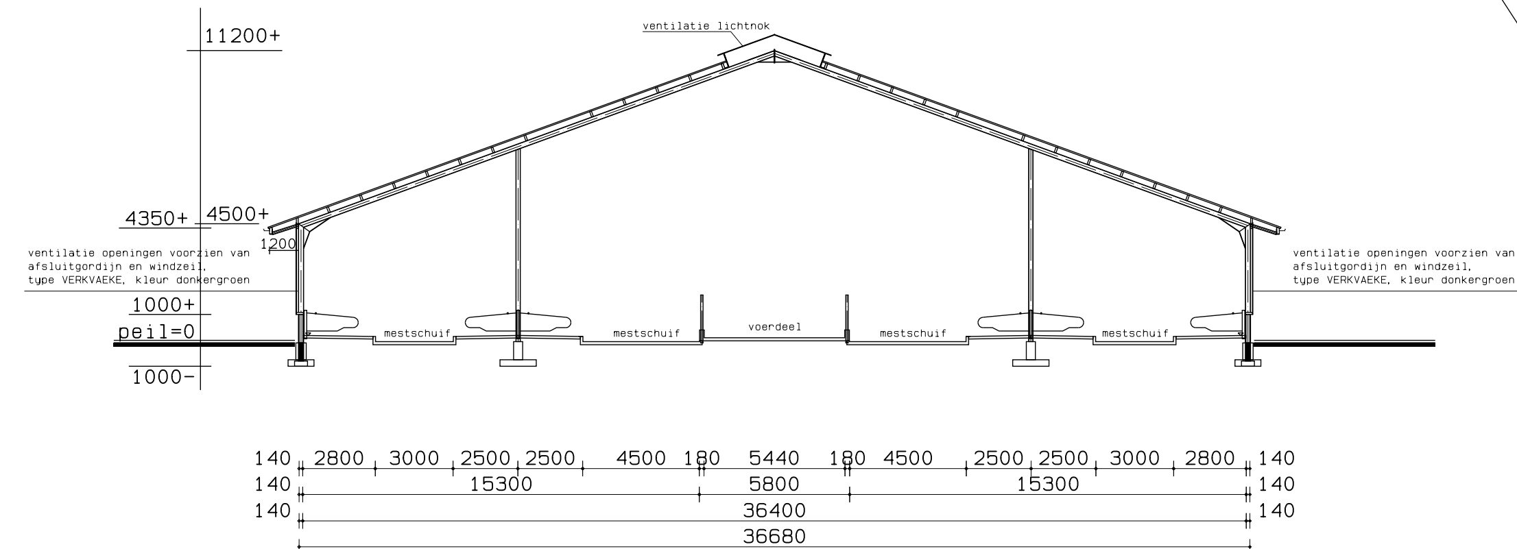
doorsnede A-A stal 1
