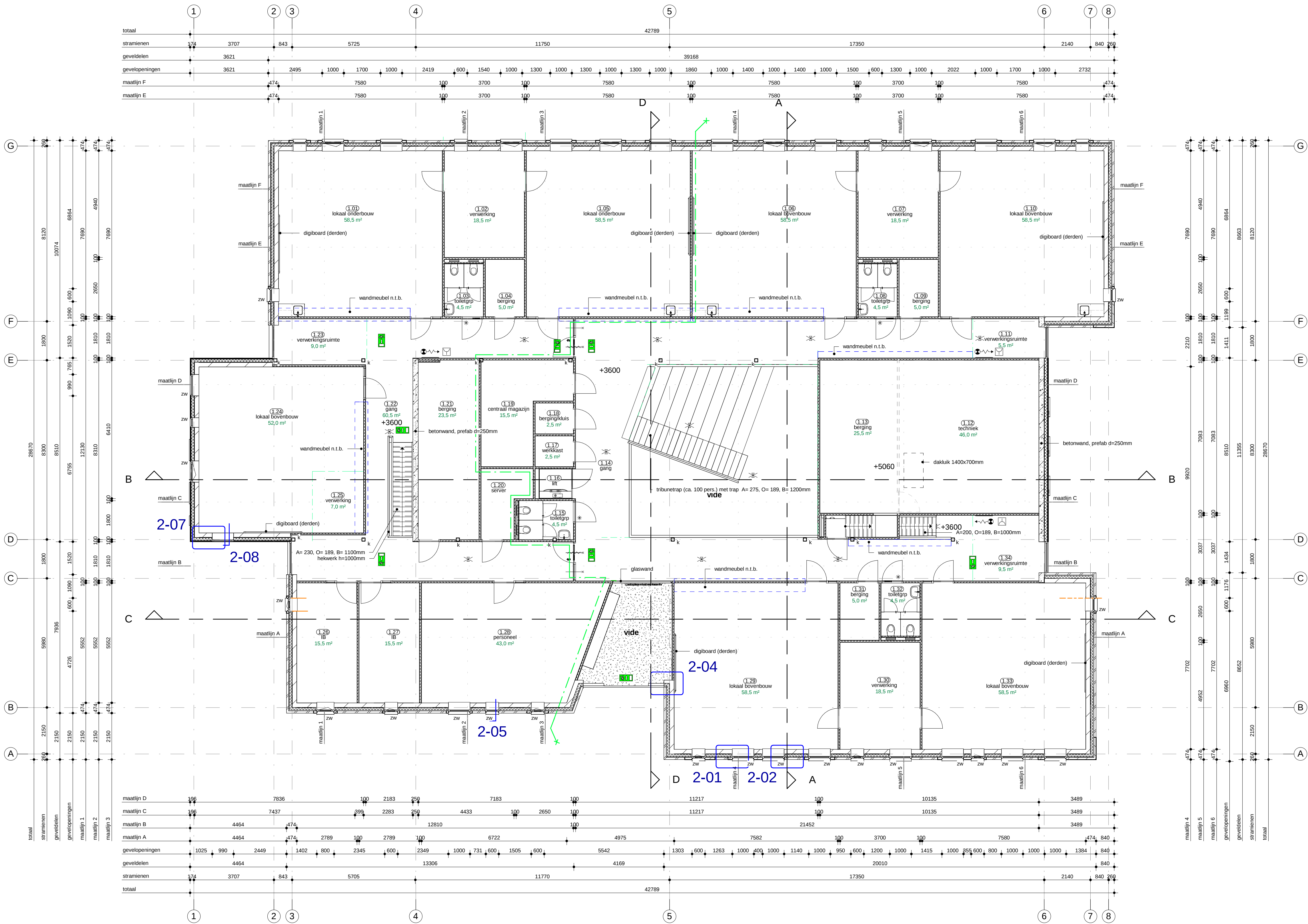
EERSTE VERDIEPING
