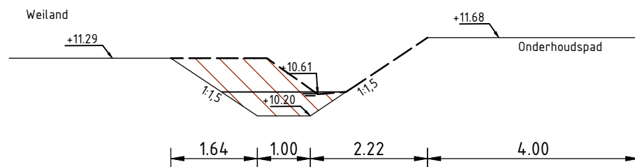
Profiel 47 Schaal 1:100
