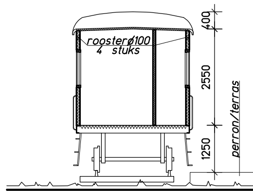
doorsnede
