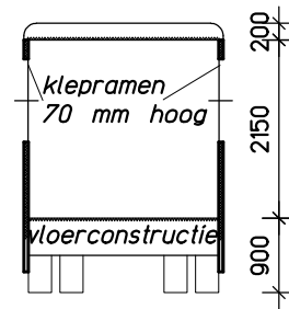
doorsnede
