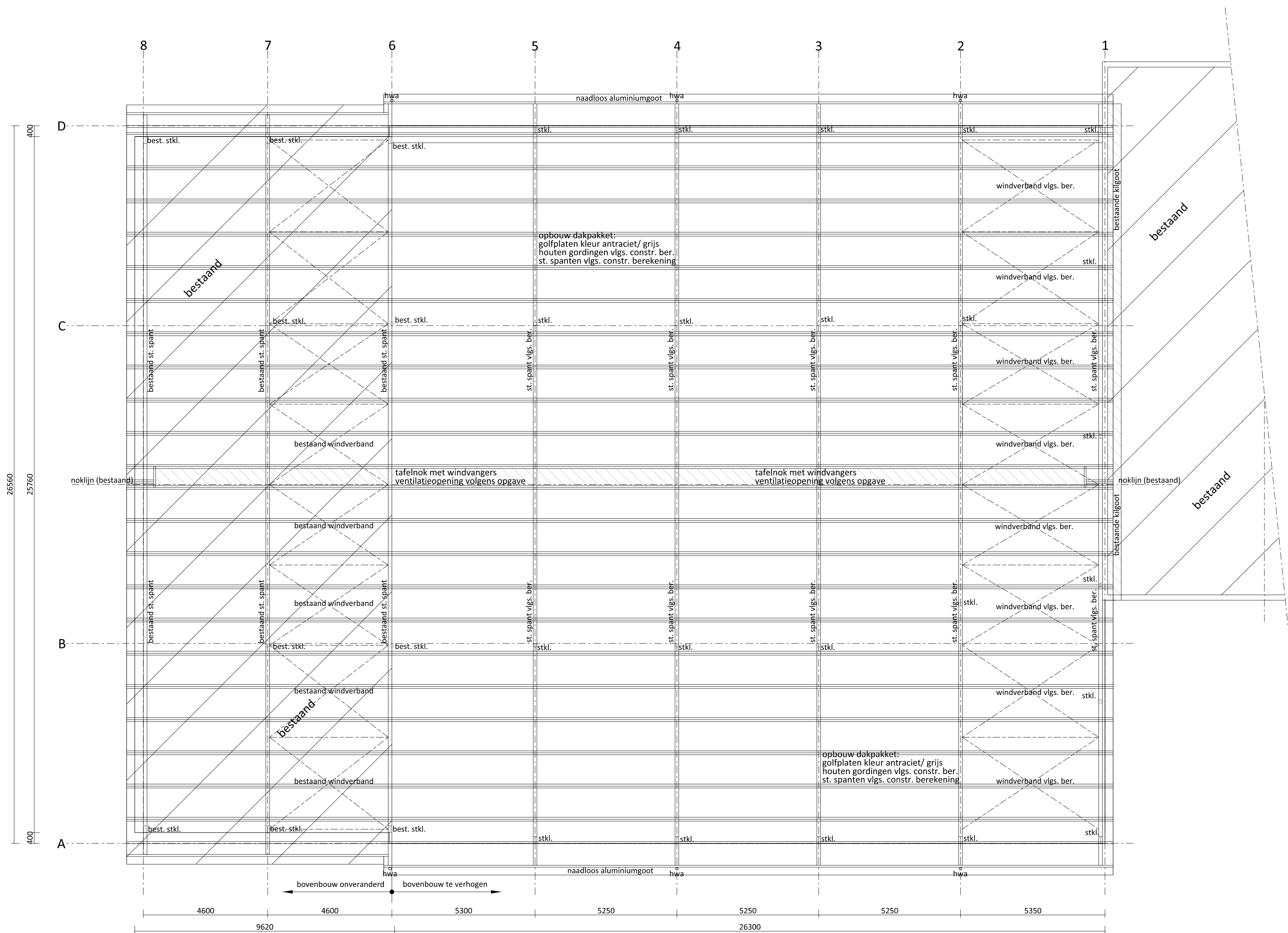
Kapplan
