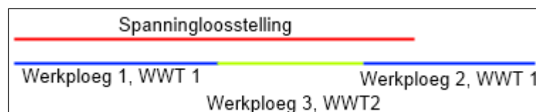
Figuur 4 - Meerdere werkploegen in gebied met spanningloosstelling
