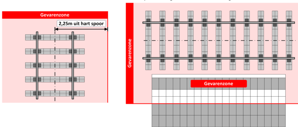
Figuur 2 - Gevaarenzone Links: vrije baan en remise
