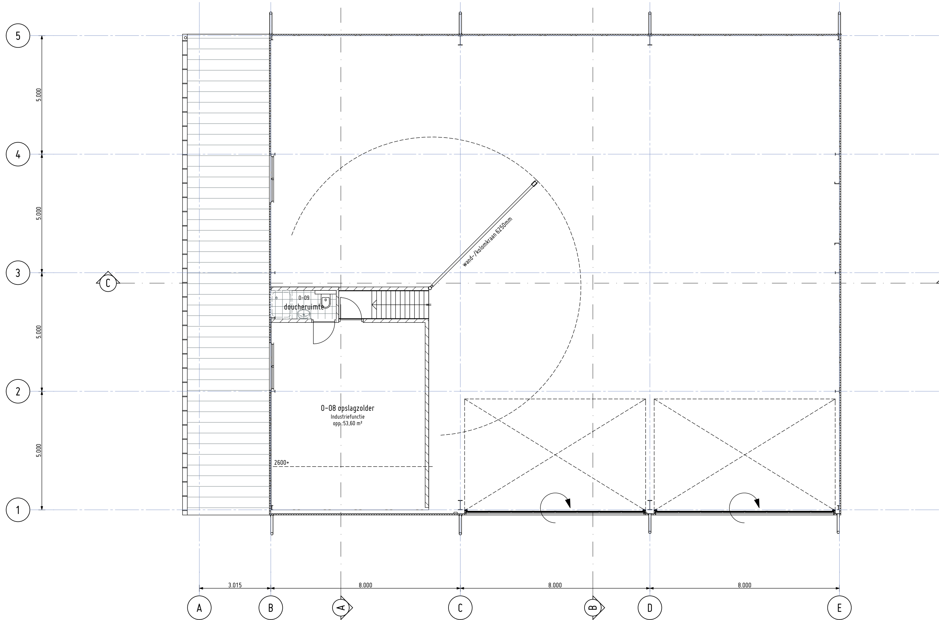
1e verdieping 1:100
