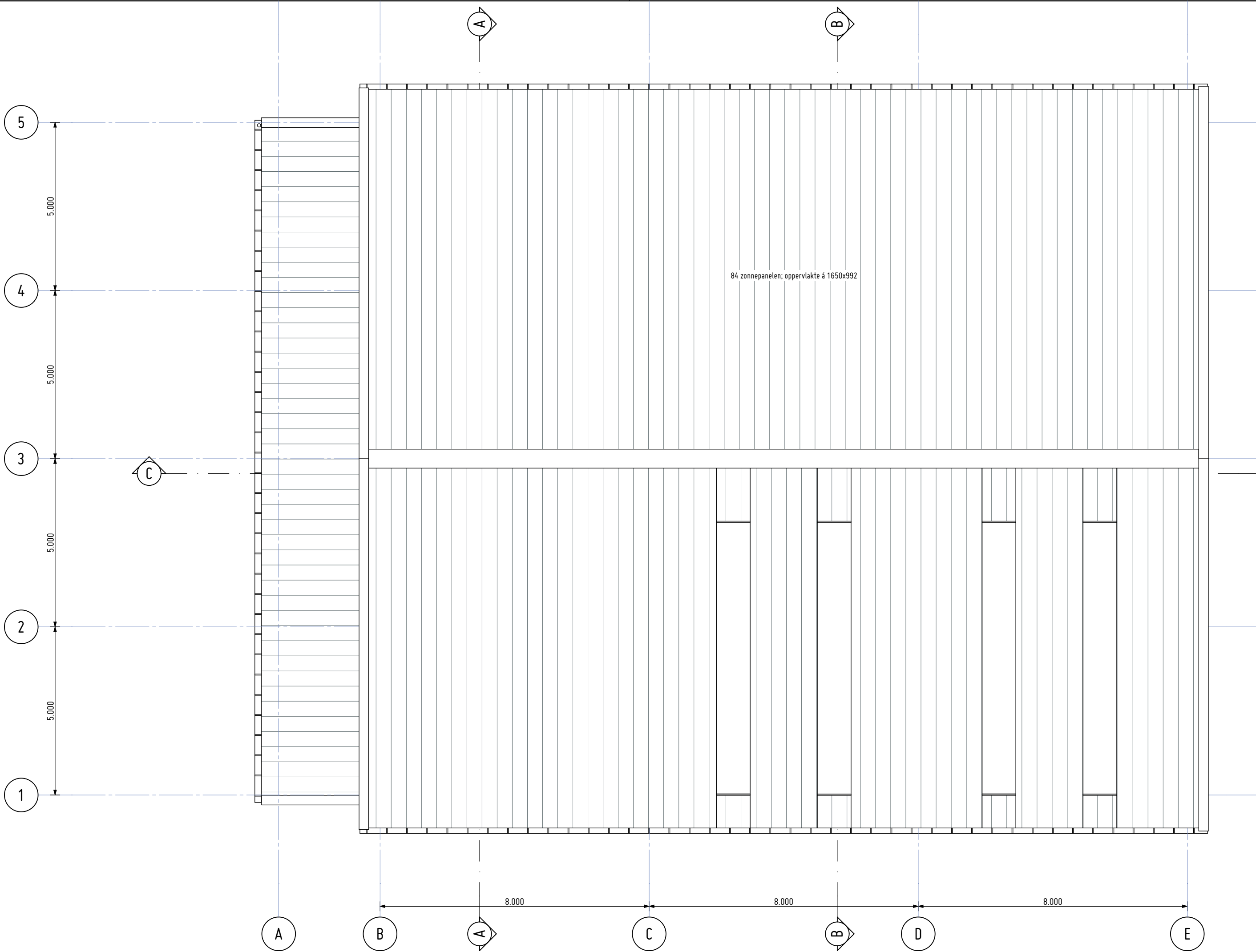
Dakoverzicht 1:100
