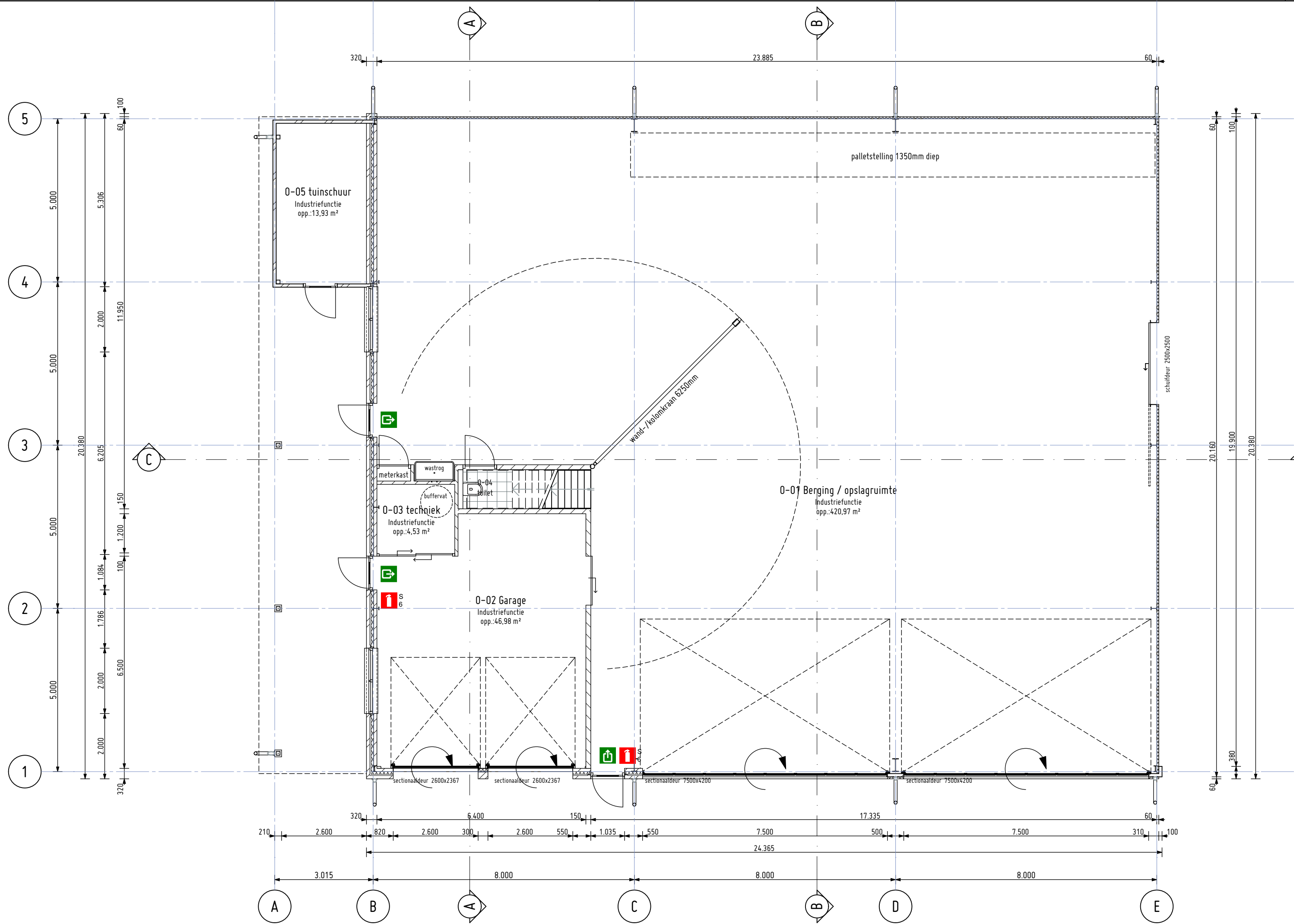
Begane grond 1:100
