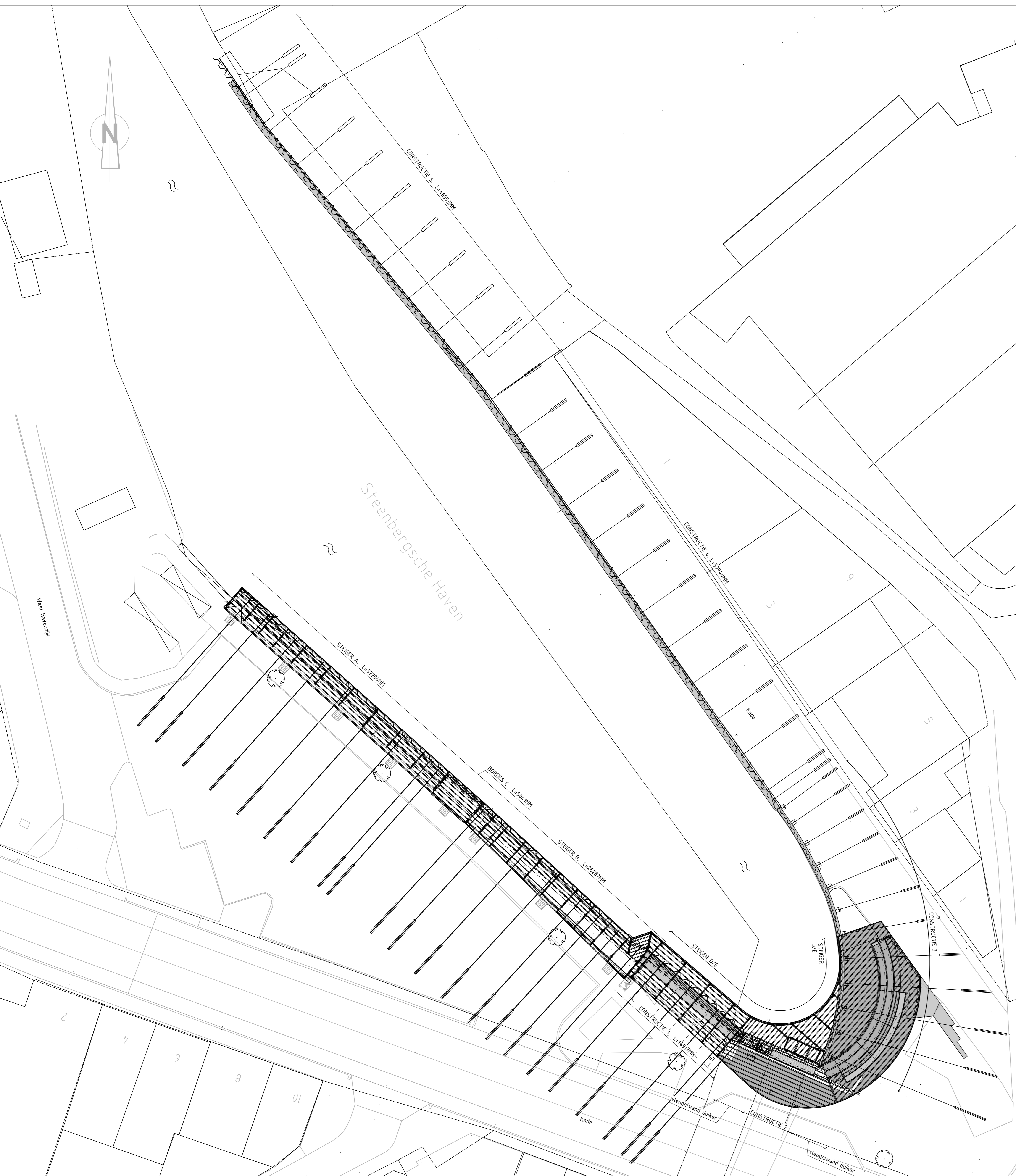
NIEUWE SITUATIE STEIGER A,B,D,E EN BORDES C SCHAAL 1:200
