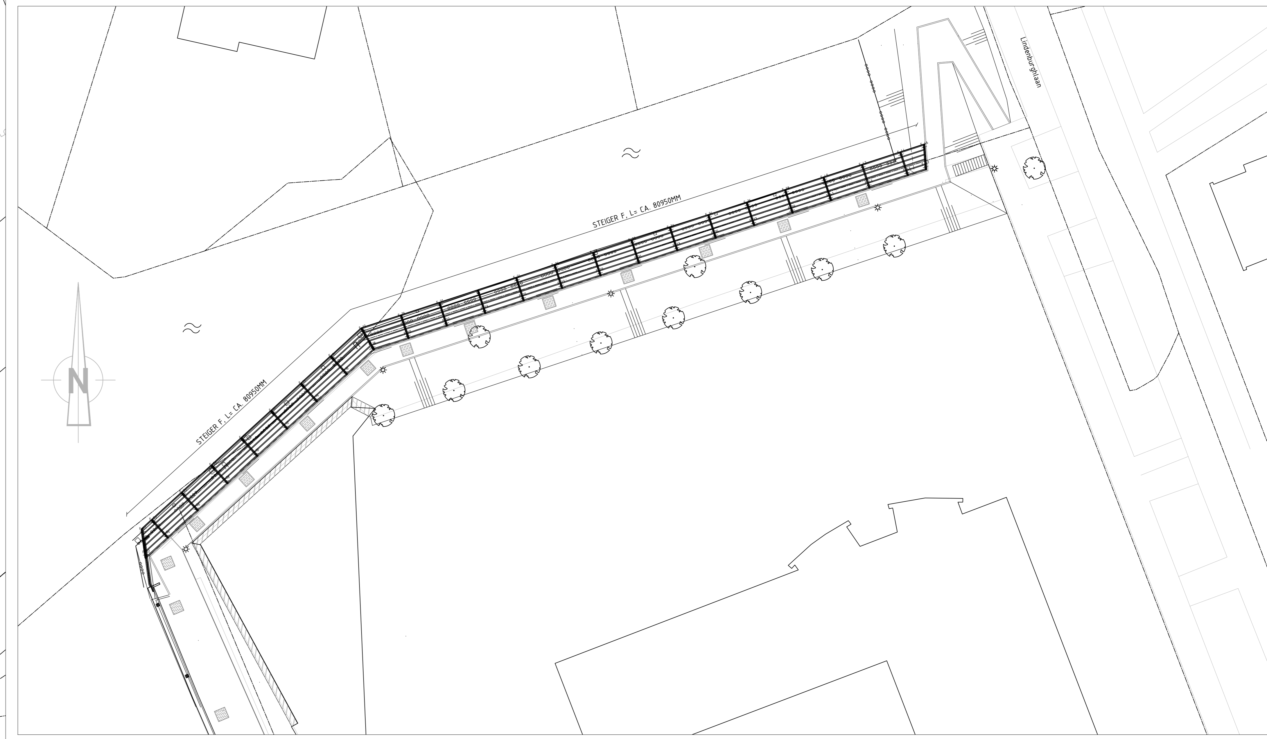
NIEUWE SITUATIE STEIGER F SCHAAL 1:200
