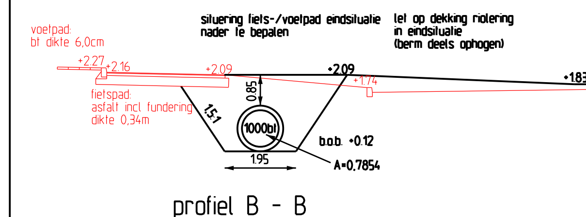
profiel B - B schaal 1:100
