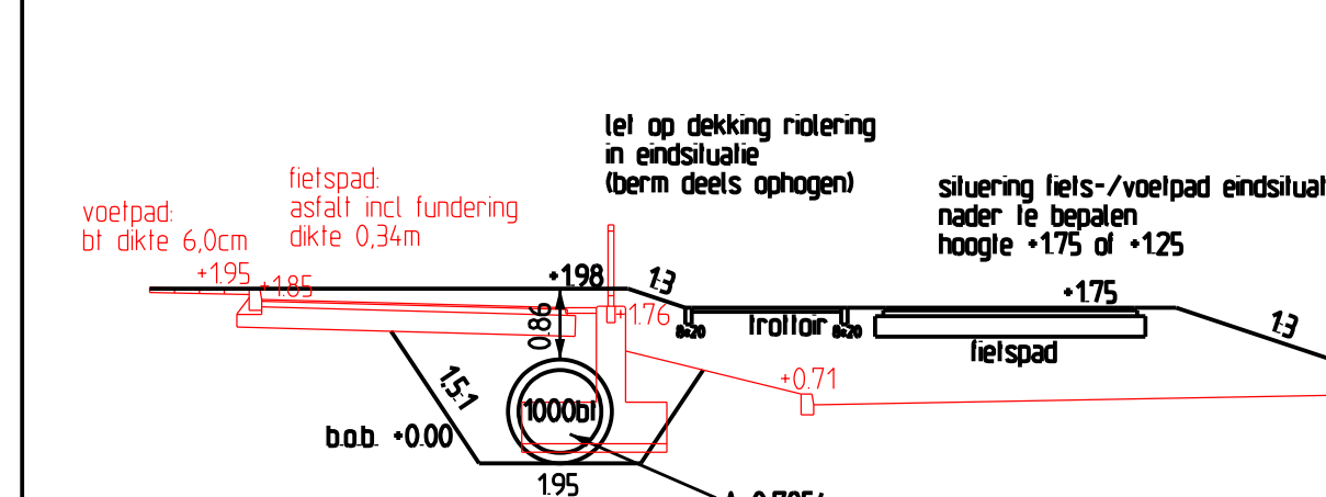
profiel C - C schaal 1:100
