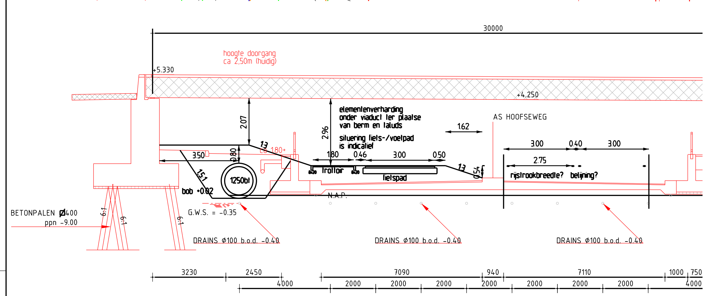
profiel D - D (hoogte doorgang fiets-/voelpad 2.96 m) schaal 1:100
