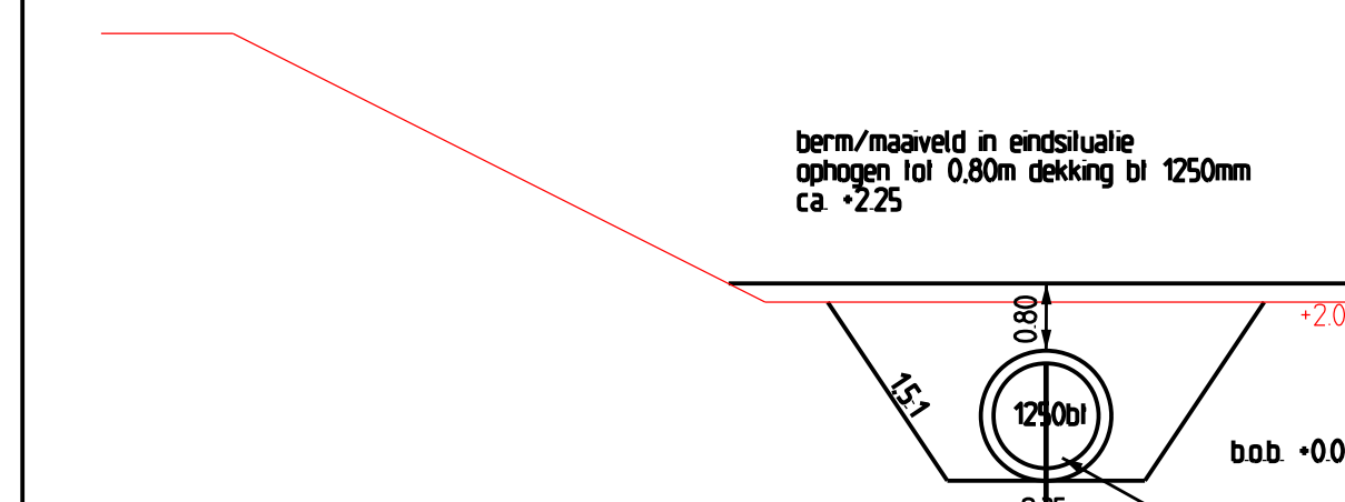
profiel E - E schaal 1:100
