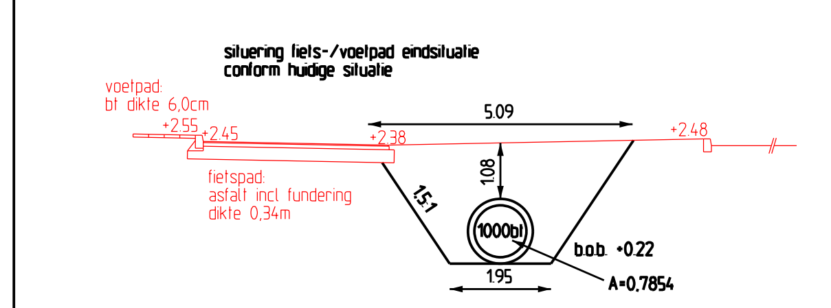
profiel A - A schaal 1:100
