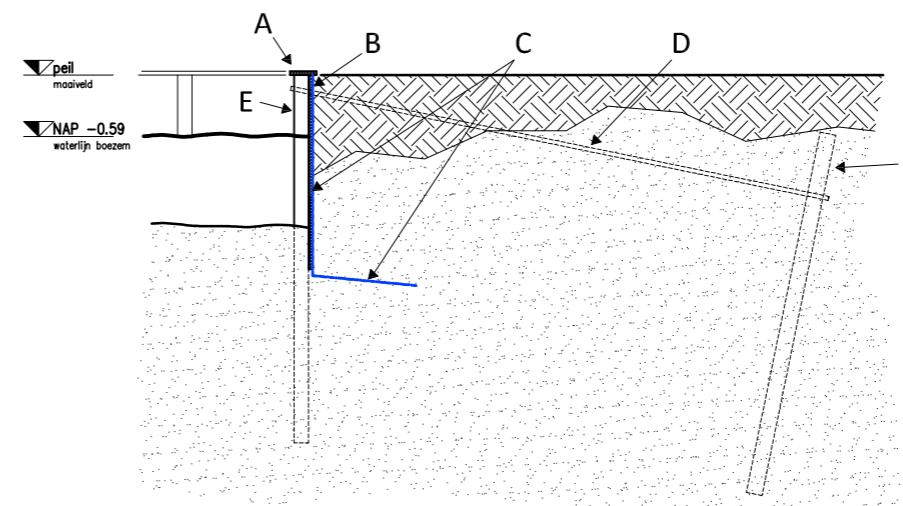
Doorsnede A - A
