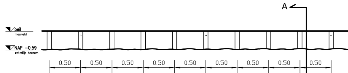
Vooraanzicht beschoeiing
