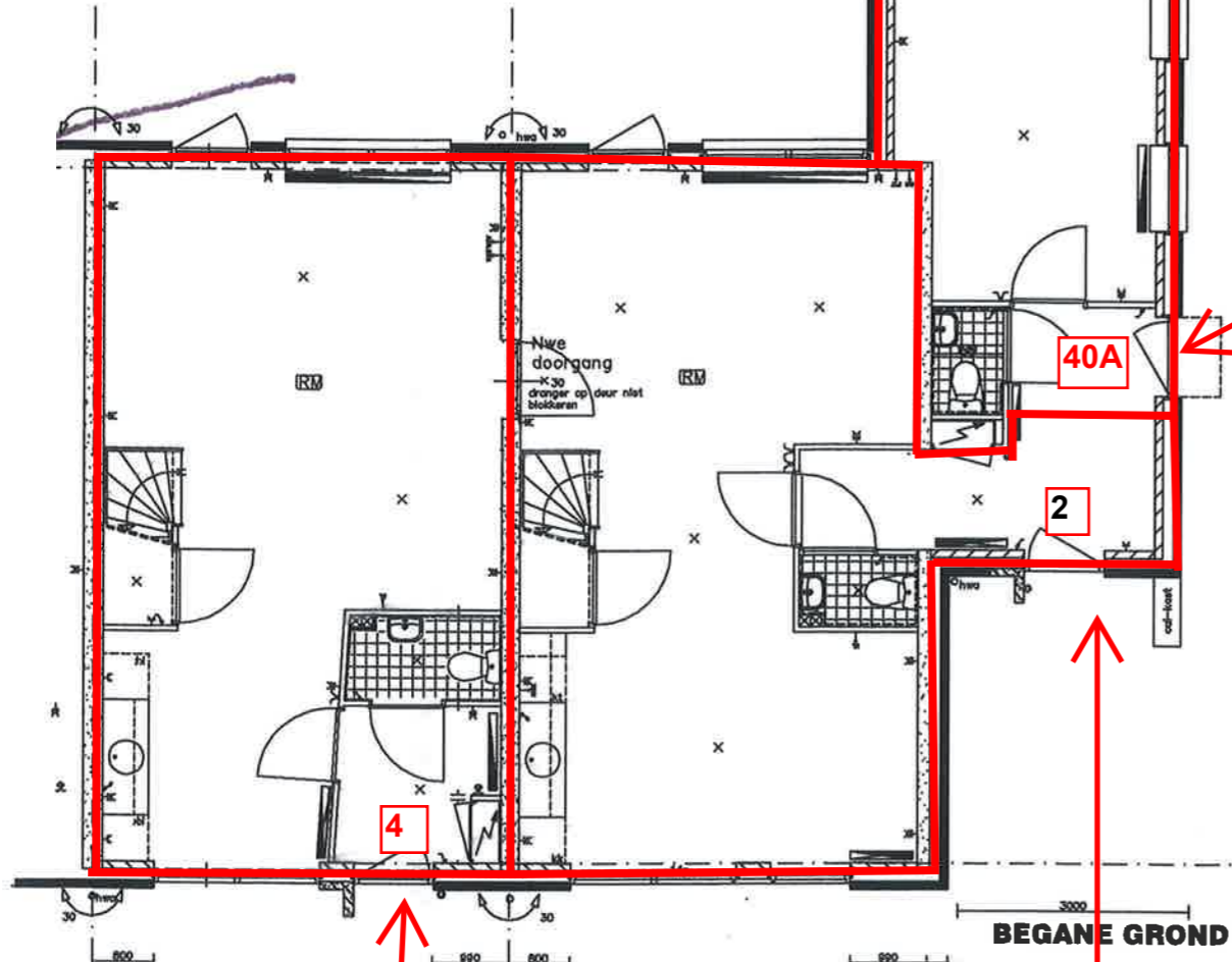
Waterbies 2, woning, begane grond, eerste en tweede verdieping
