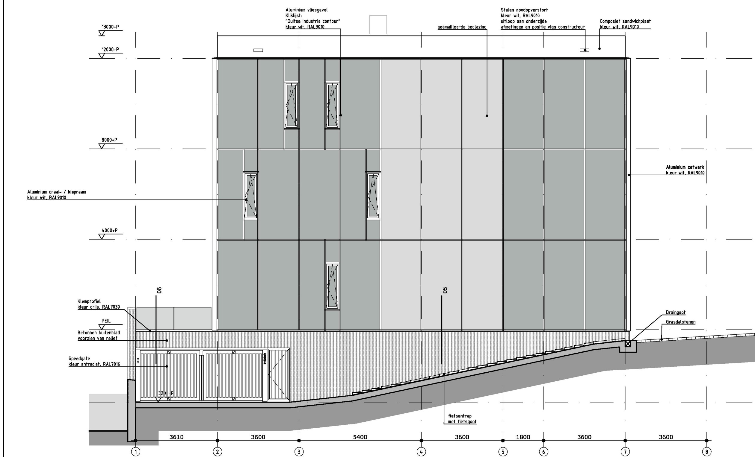
Zijgevel links / Doorsnede F - F
