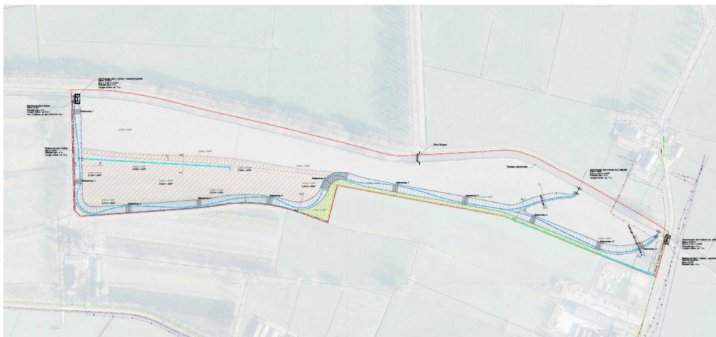
Kaart ontwerp vispassage rond stuw Rutgers
