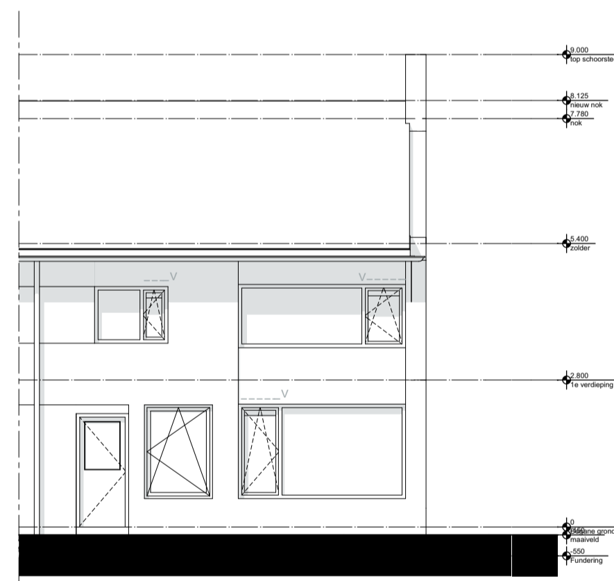
Achtergevel 1/100
