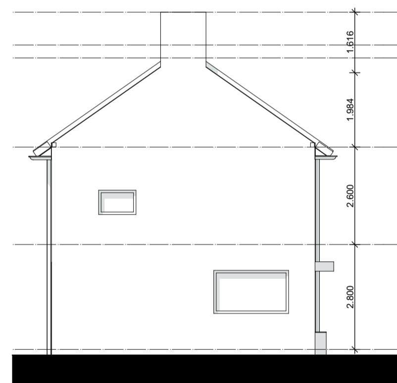
Linkergevel 1/100
