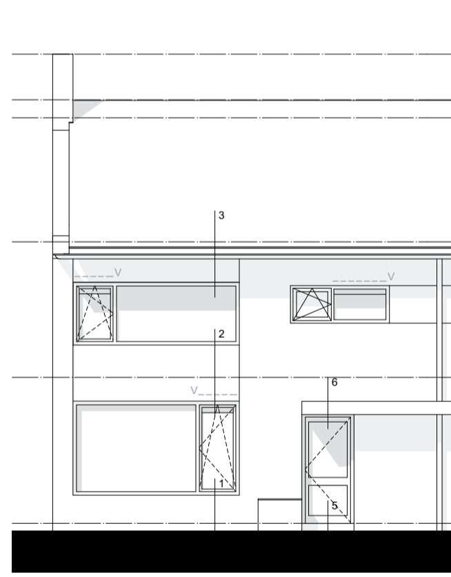
Voorgevel 1/100
