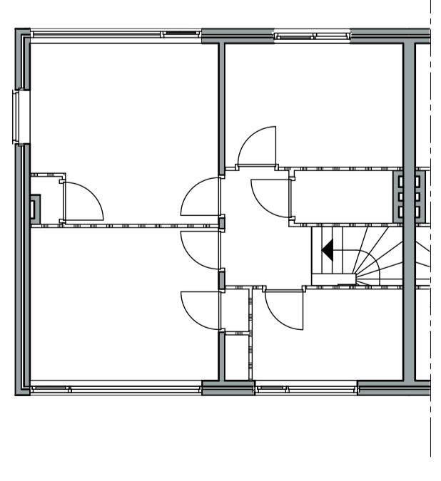
1e verdieping
