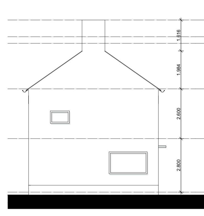
Linkergevel
