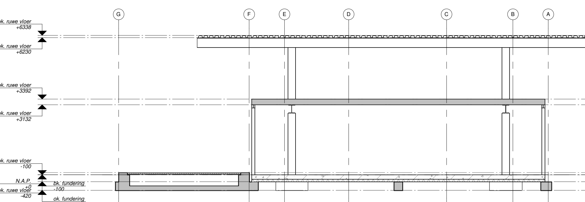
Principe doorsnede 4
