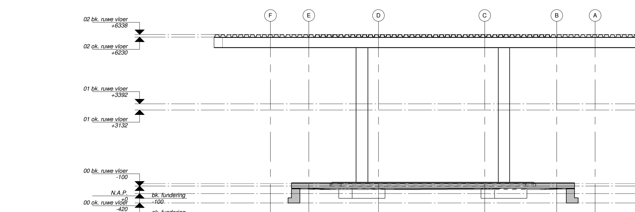
Principe doorsnede 6
