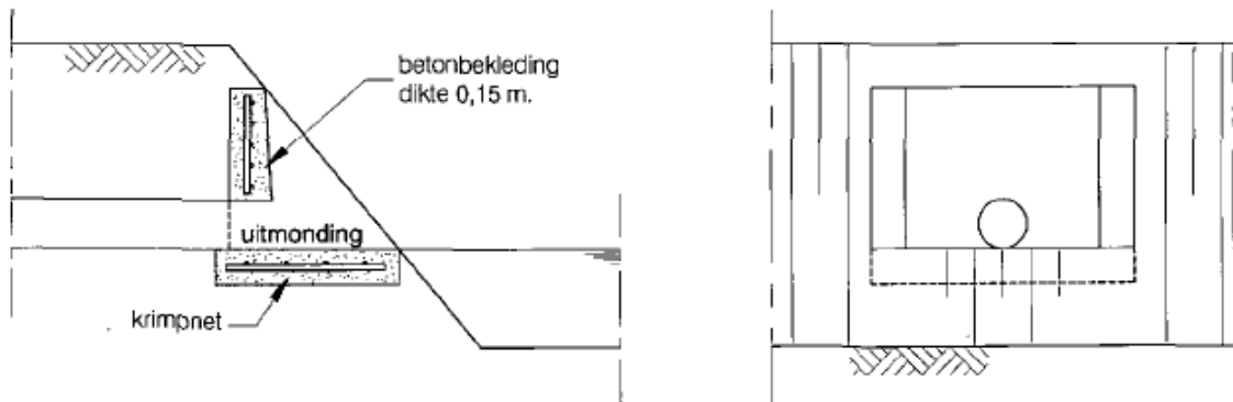
Dwarsdoorsnede A-A
