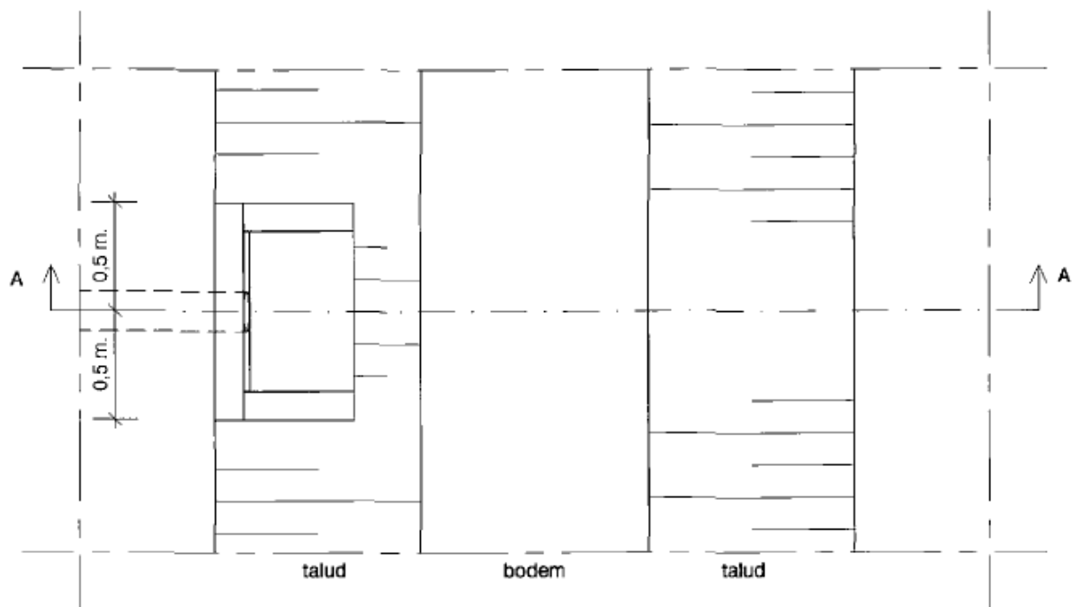
Bovenaanzicht
