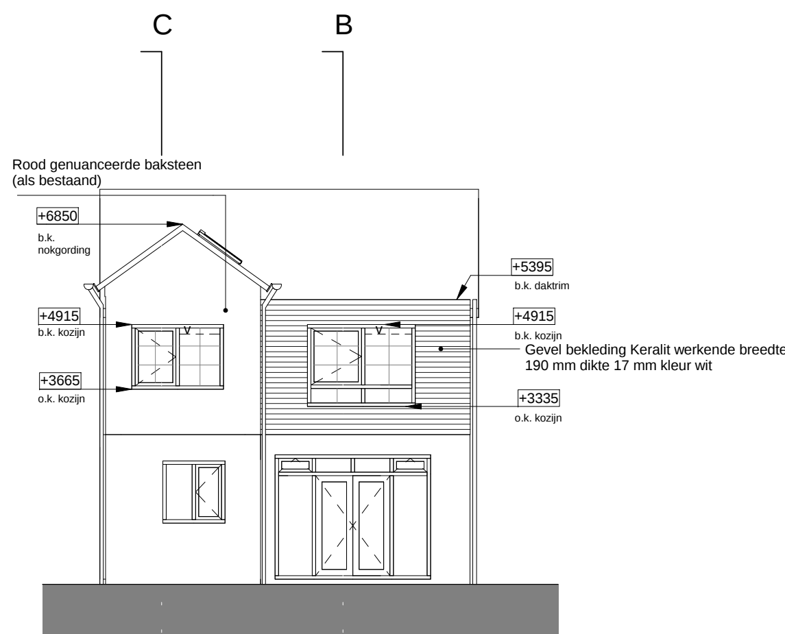
Achter aanzicht
