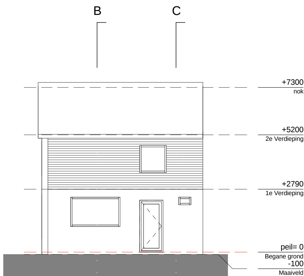
Vooraanzicht - ongewijzigd
