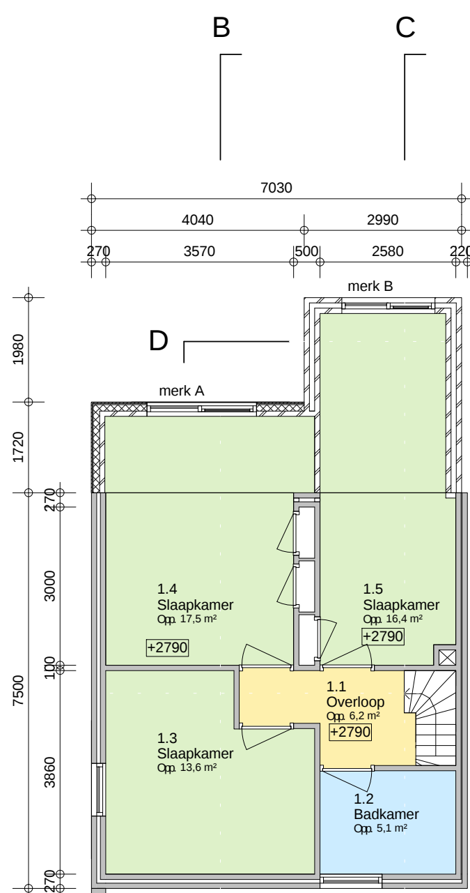
1e Verdieping
