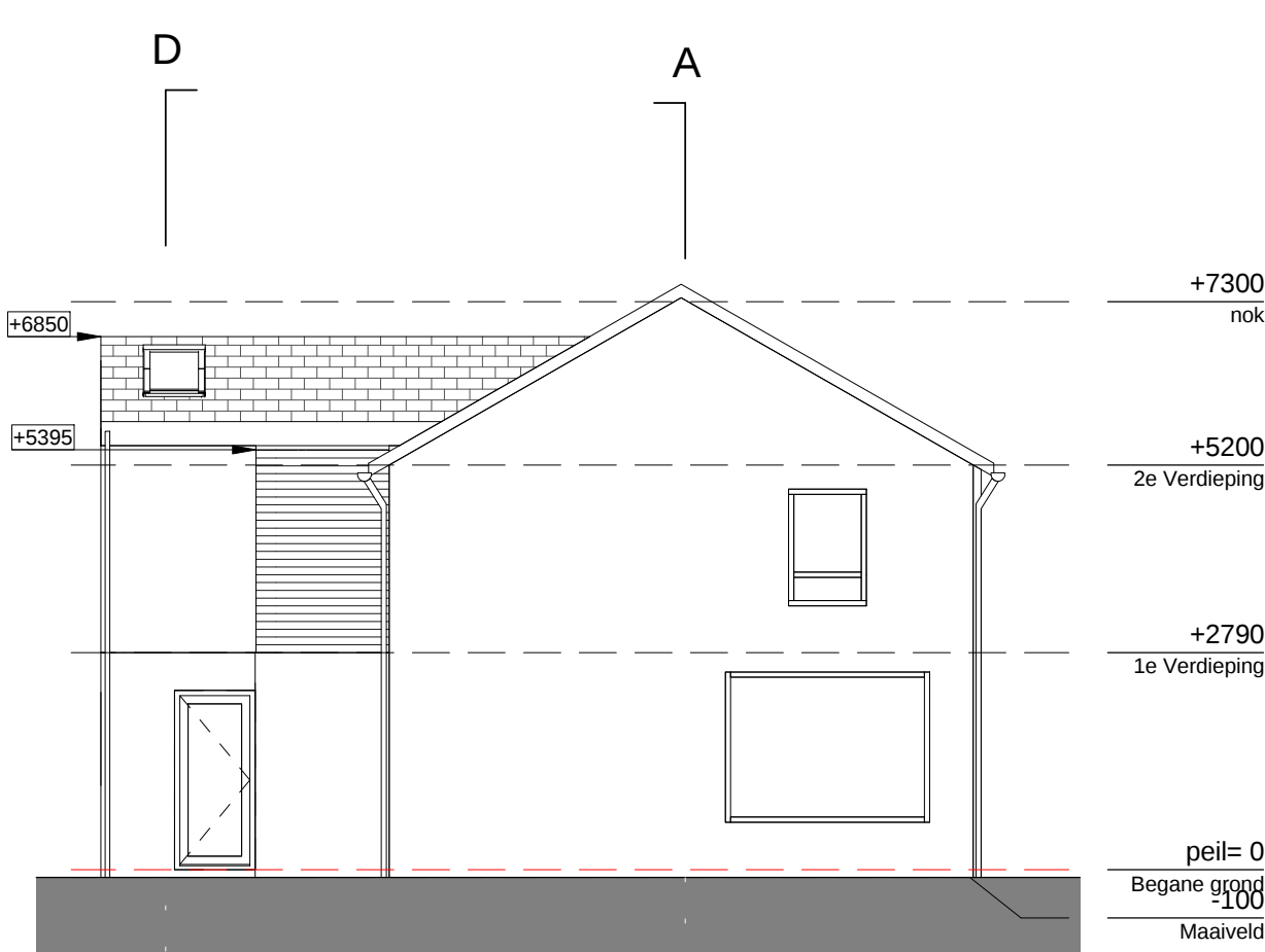
Linker aanzicht
