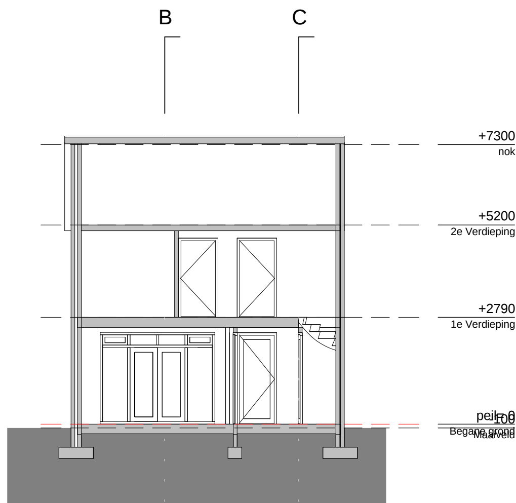
Doorsnede A
