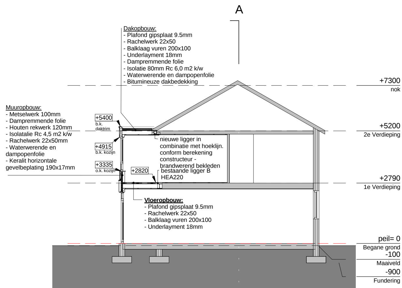
Doorsnede B
