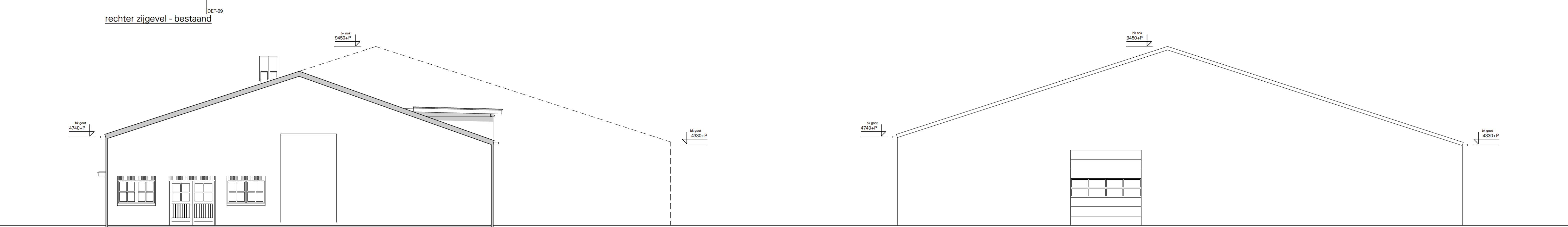
achtergevel - bestaand
