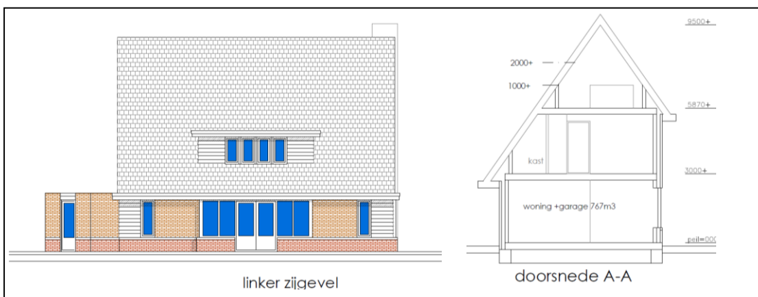
afb. 13 aanzicht zijgevel en doorsnede
