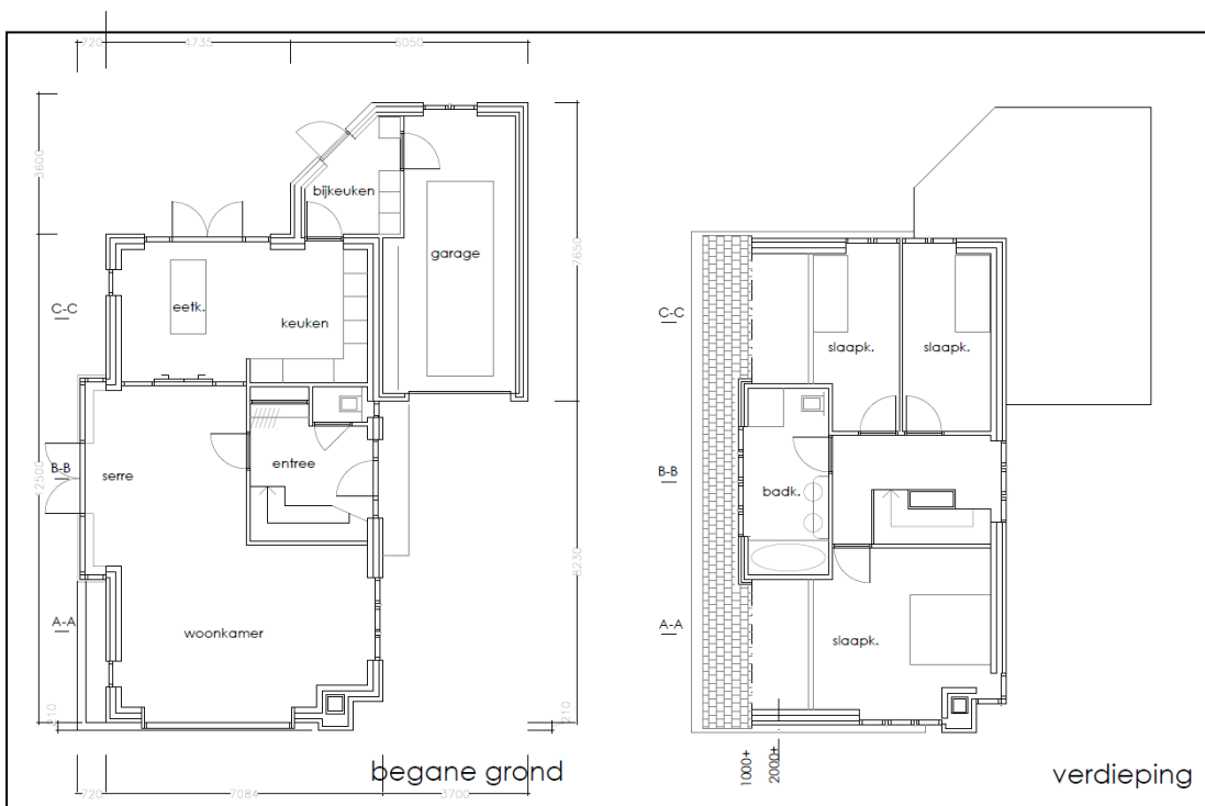
afb. 12 De plattegrond van begane grond en de verdieping
