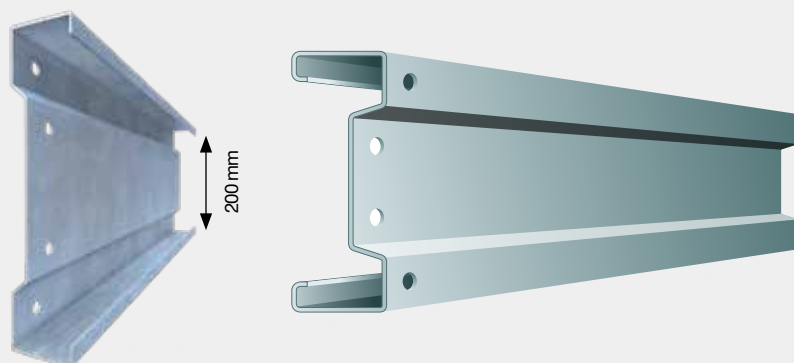
Constructieprofiel Sigma 200+
