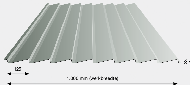
Potdekselprofielplaat 23/1000
