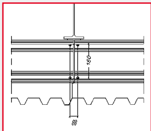
Regel voor spanten langs (op strip)
