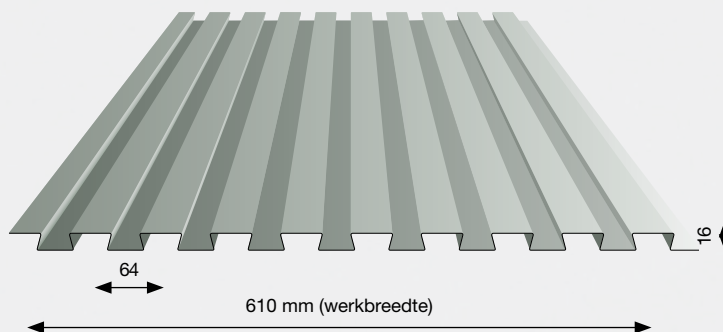
Zwaluwstaartprofielplaat 16/610
