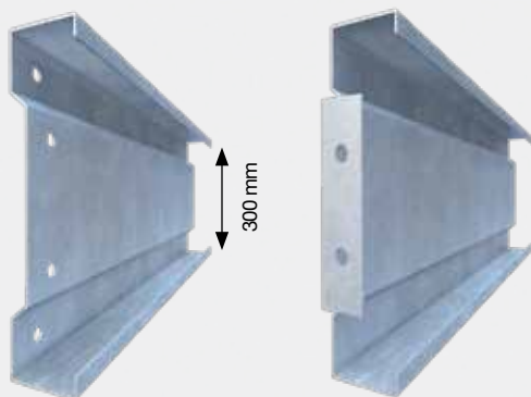
Constructieprofiel Sigma 200 - 230 - 300 - 400
