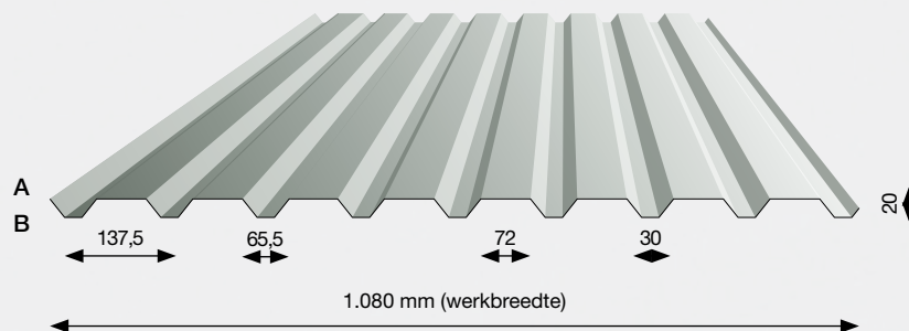
Damwandprofielplaat 20/1080
