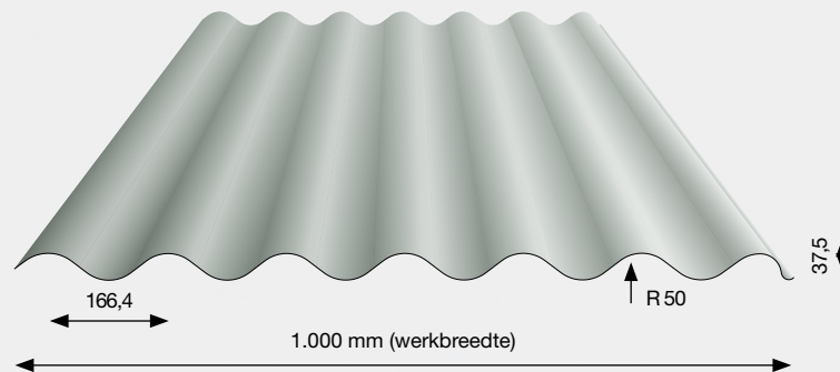
Golfprofielplaat 38/1000
