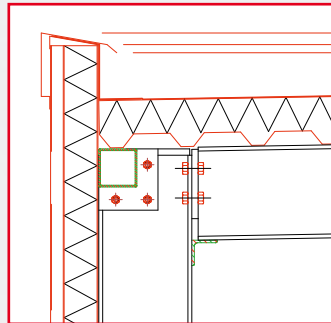
Platdak dakrand
