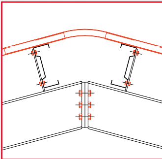
Profielplaat nok
