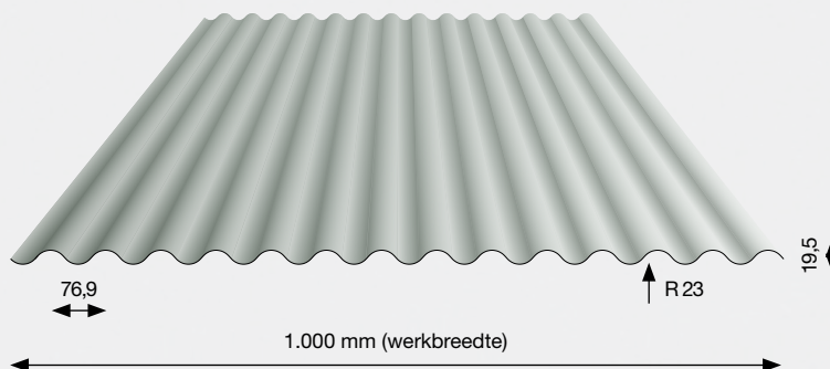
Sinusplaat 20/1000
