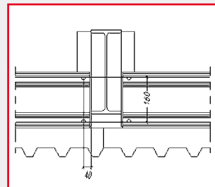
Regel tussen spanten (op hoeklijn)
