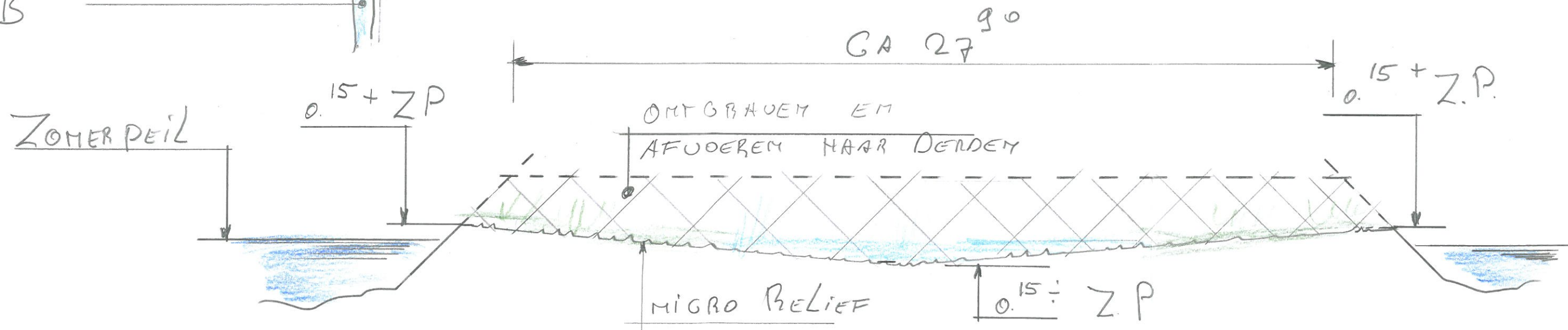
DWARS PROFIEL B-B
