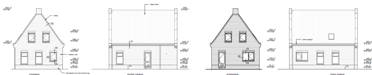
4. Afbeelding: Bouwtekening woning
