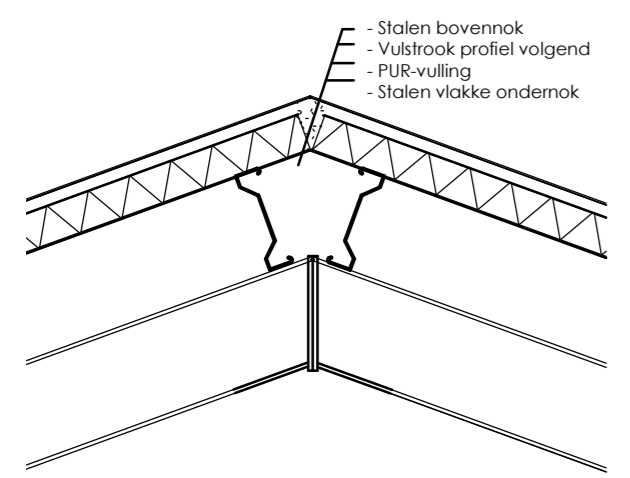
Doorsnede A-A 1:50
