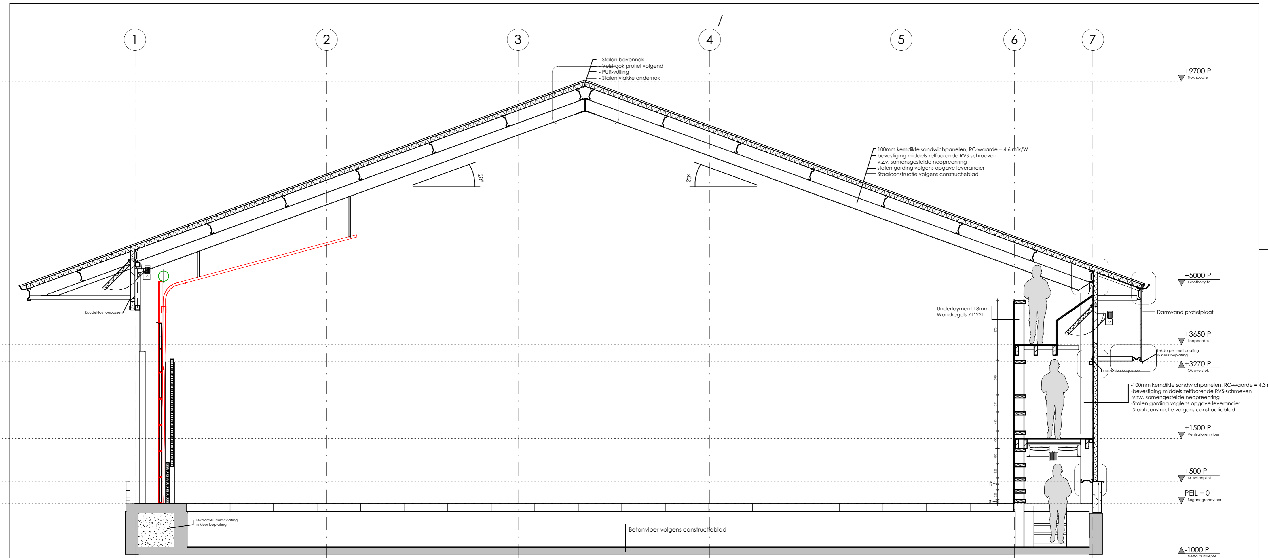
Doorsnede A-A 1:50
