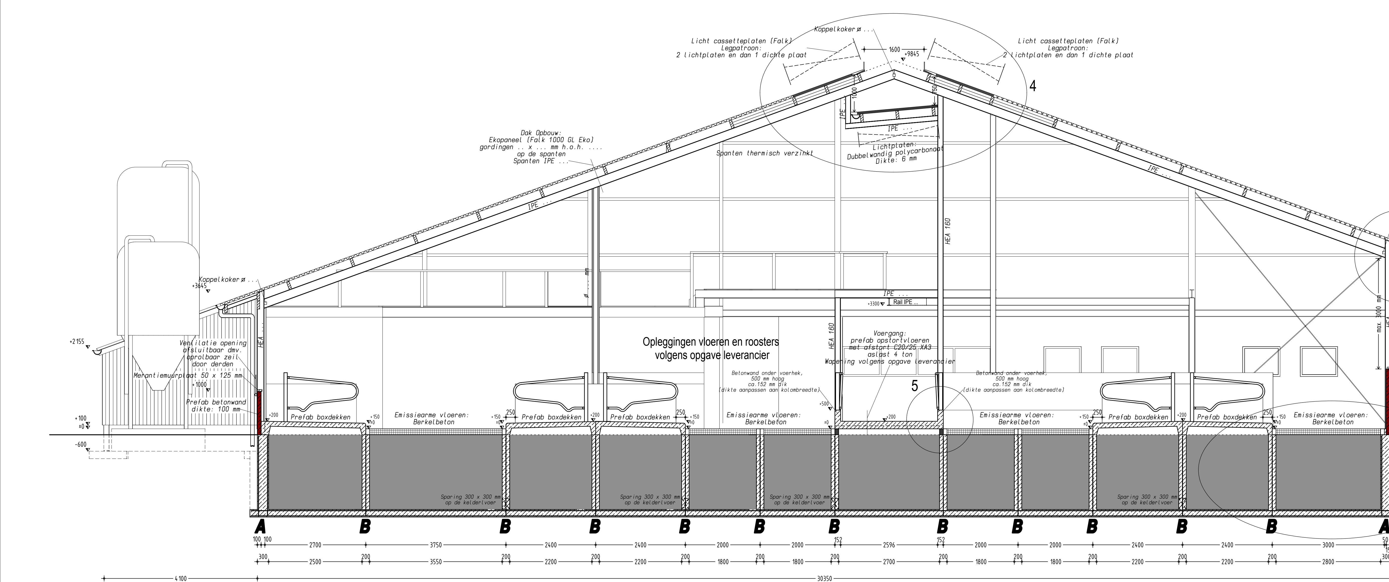
Doorsnede B-B
