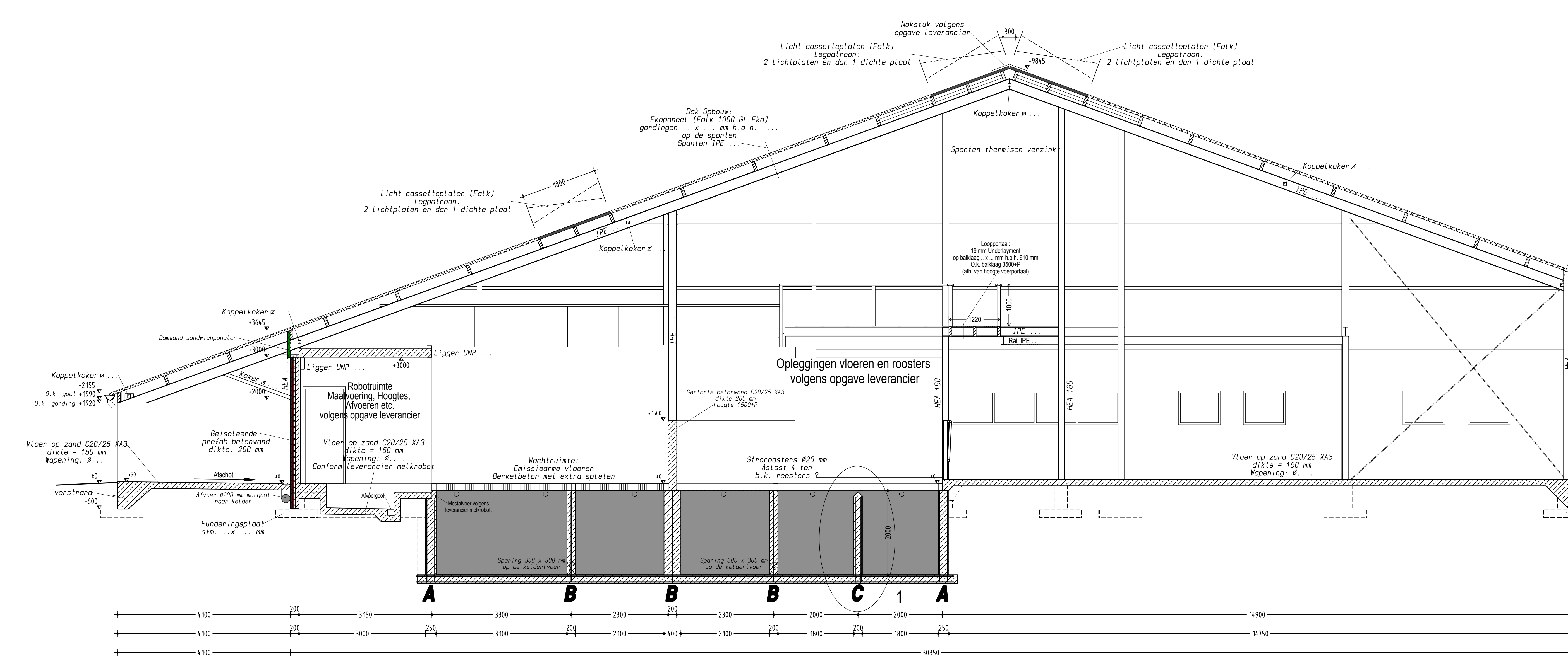
Doorsnede A-A
