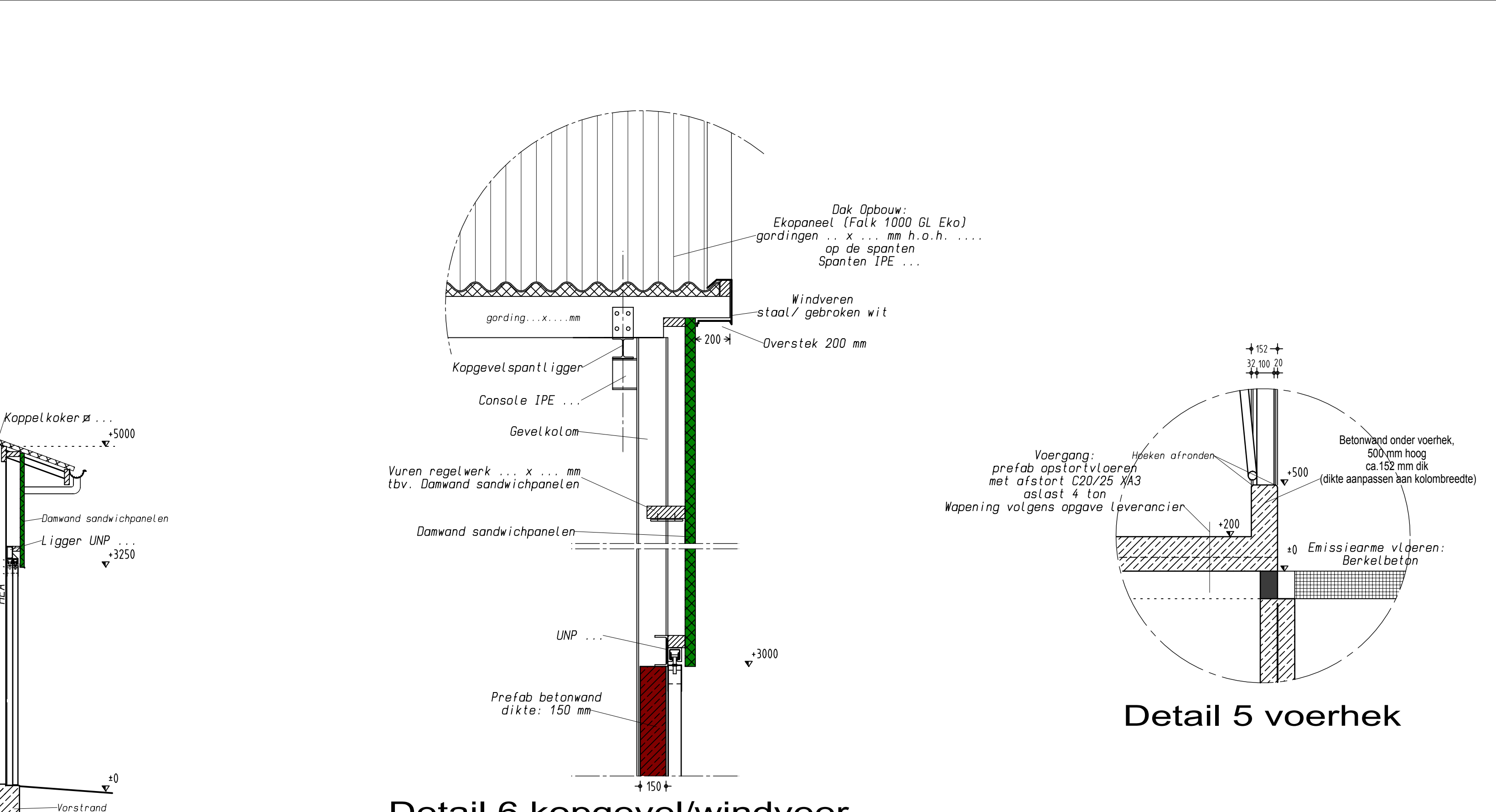
Detail 5 voerhek
