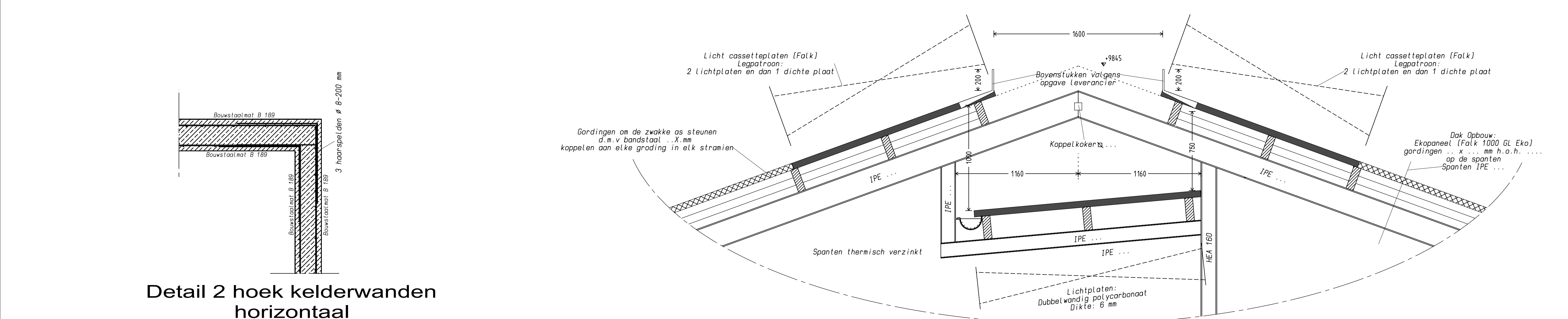
Detail 2 hoek kelderwanden horizontaal
