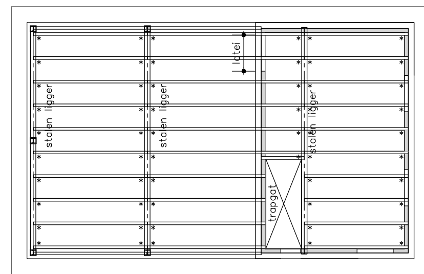
balklaag
