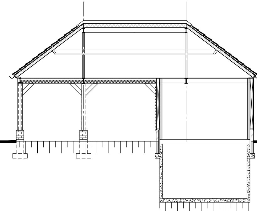
langsdoorsnede
