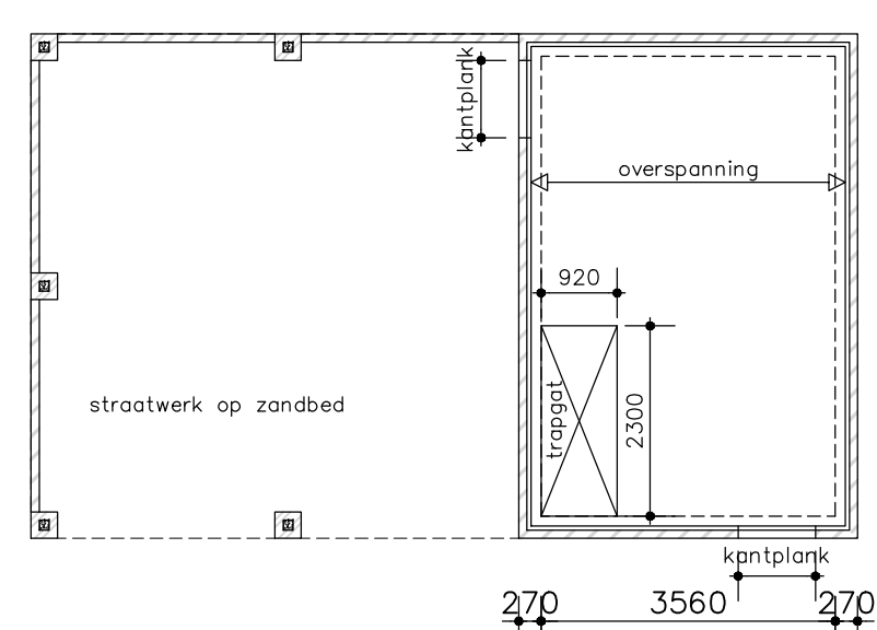
beganegrondvloer
