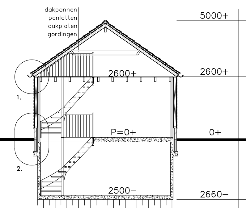
dwarsdoorsnede
