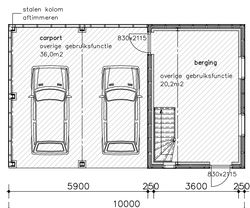
plattegrond
