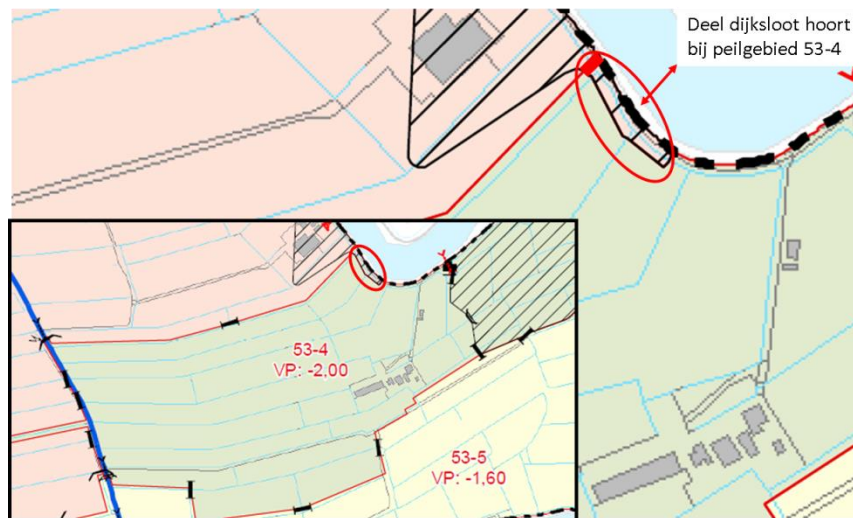
Figuur: Uitsnede concept ontwerp watergebiedsplan Hoeker en Garstenpolder en aanpassing begrenzing peilgebied 53-3 en 53-4.
