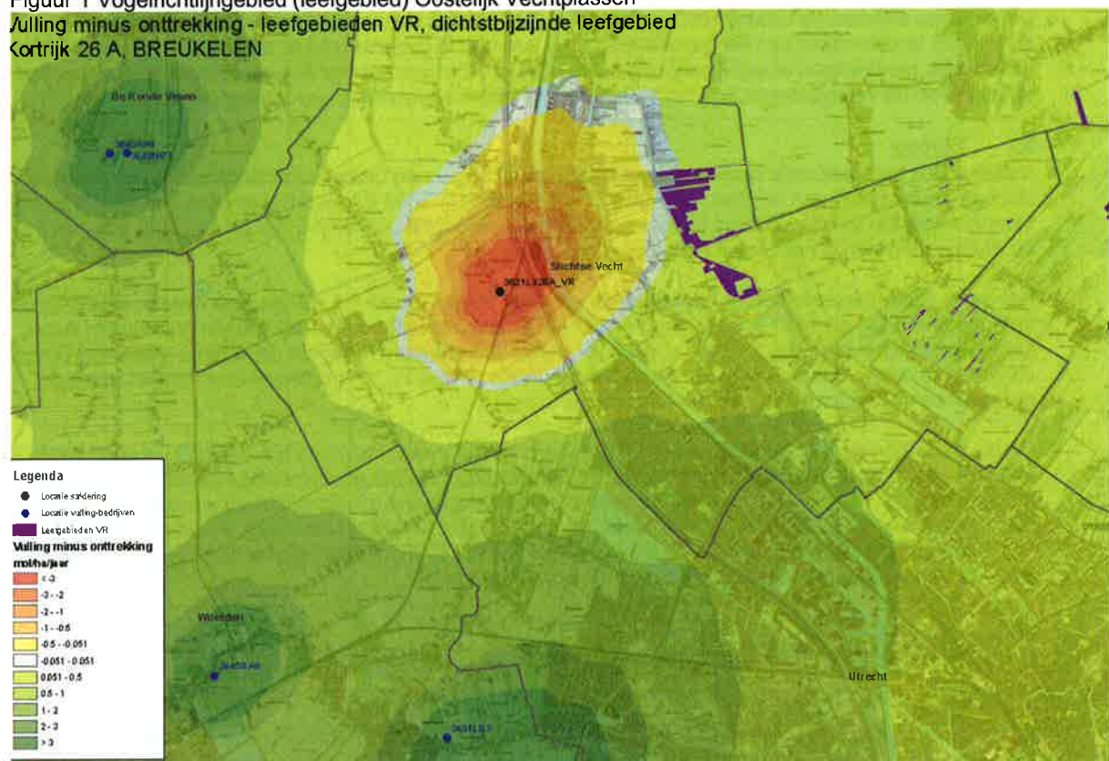
Figuur 1: Verdeling toe- en afnames van stikstofdepositie als gevolg van de toegepaste saldering voor Kortrijk 26a te Breukelen. Rood tot en met geel betreffen toenames en de groene kleuren betreffen afnames. Het witte gebied betreft een waarde tussen -0,051 en +0,051 mol N/ha/jr.
