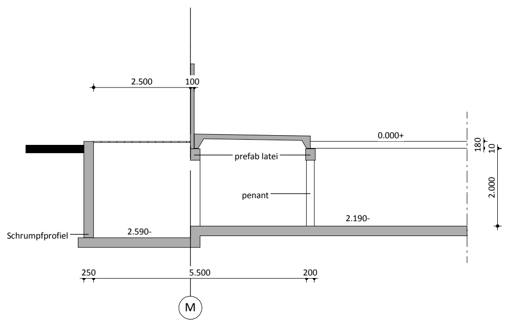
doorsnede pompputten
