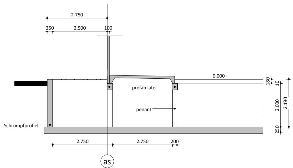
doorsnede pompput
