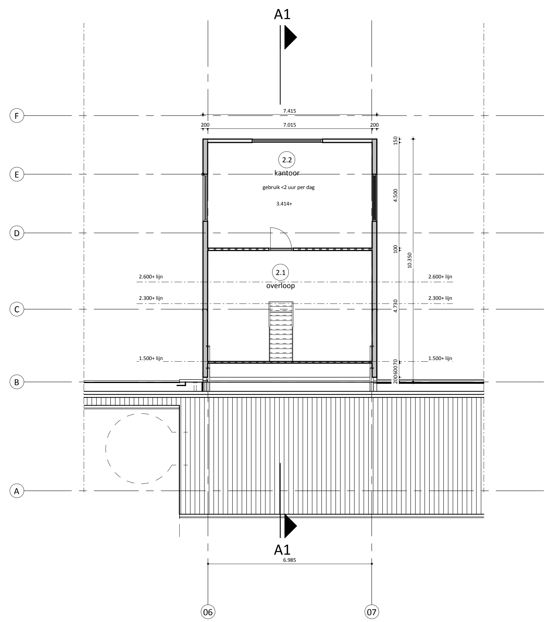
verdieping
