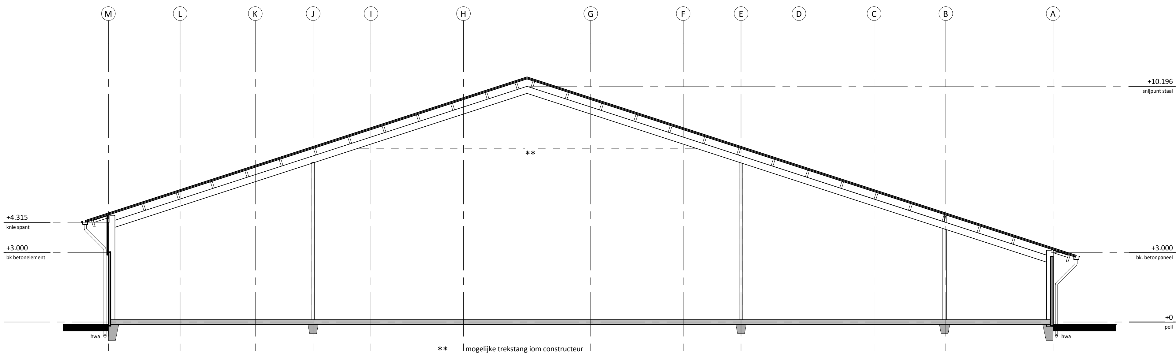
doorsnede A2
