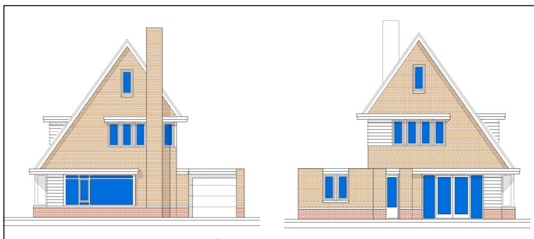
afb. 11 gevelaanzicht wegzijde en tuinzijde
