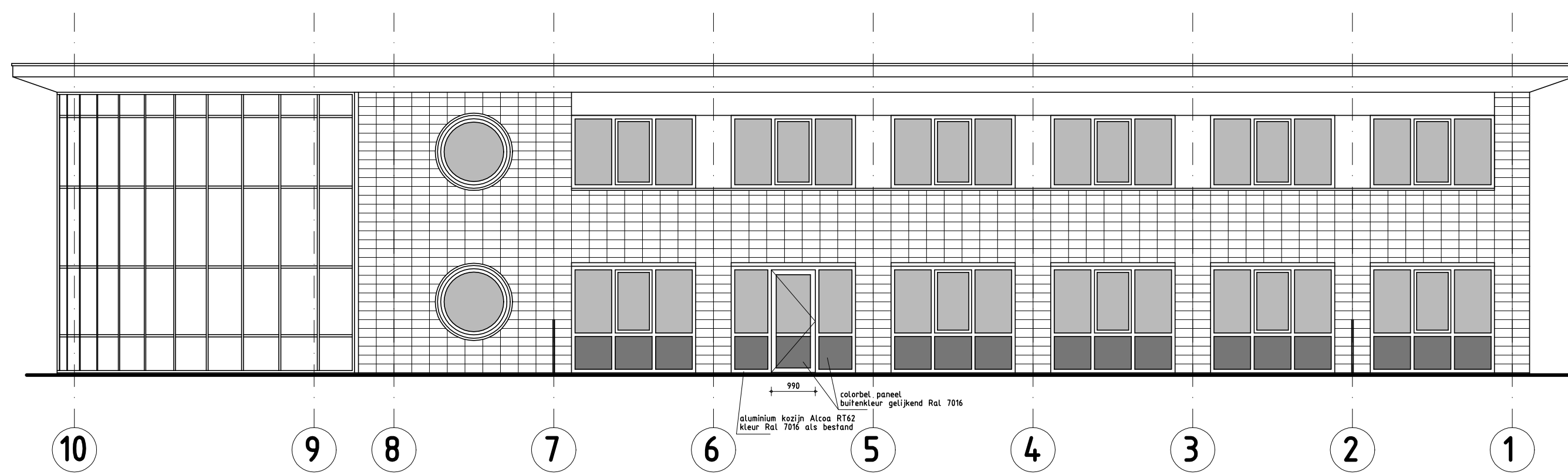
straatgevel stramen D (gewijzigd)
