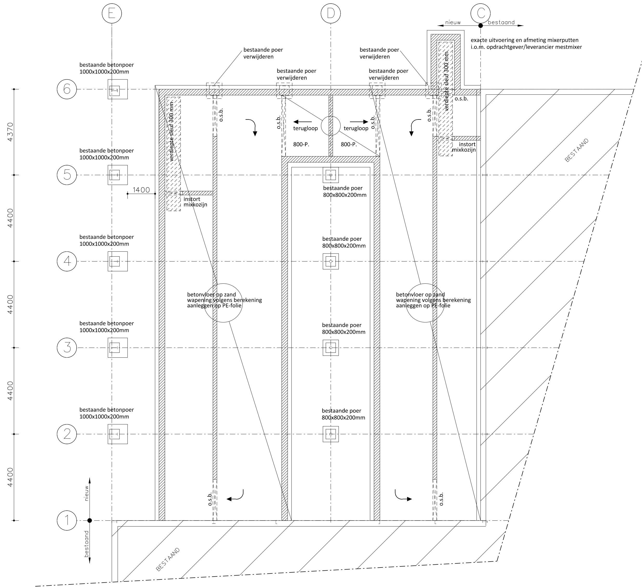
Kelder-/funderings-/ vloerenplan
