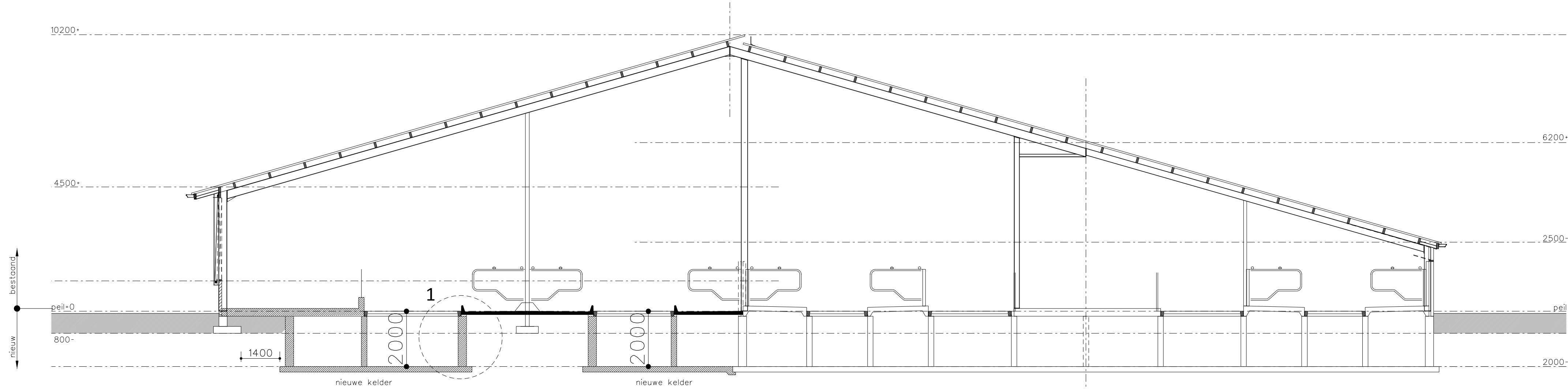
Doorsnede A-A
