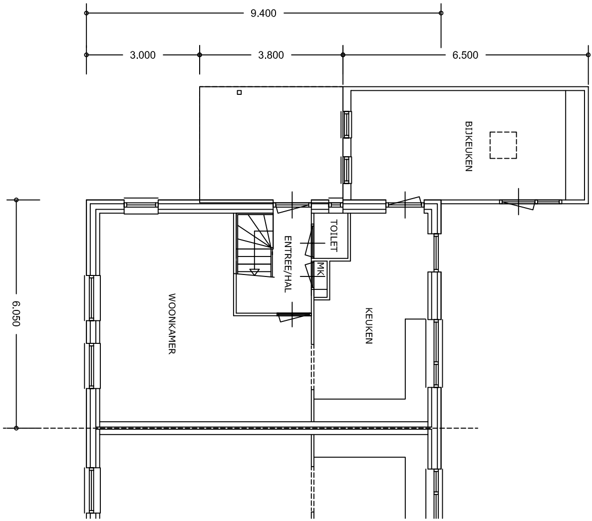
BEGANEGROND
