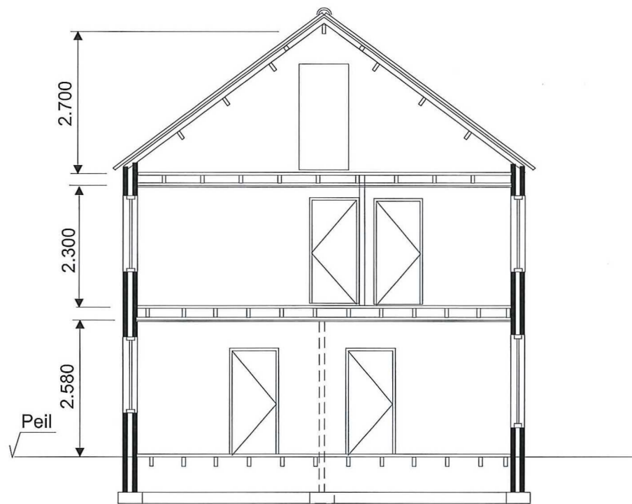
Doorsnede A - A Bestaande situatie
