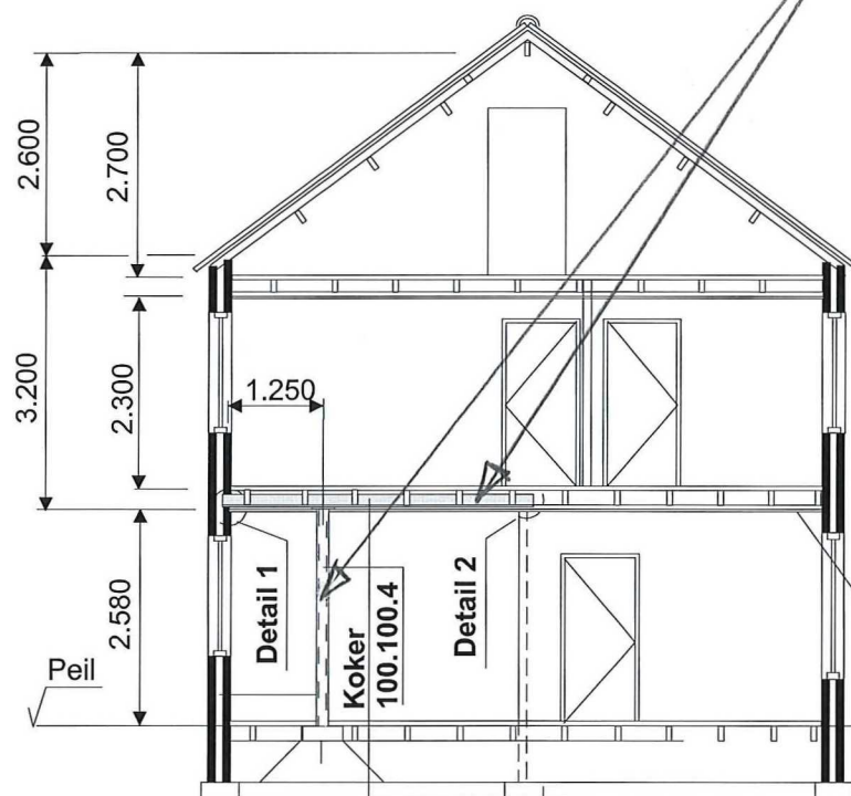
Doorsnede A - A Gewijzigde situatie
